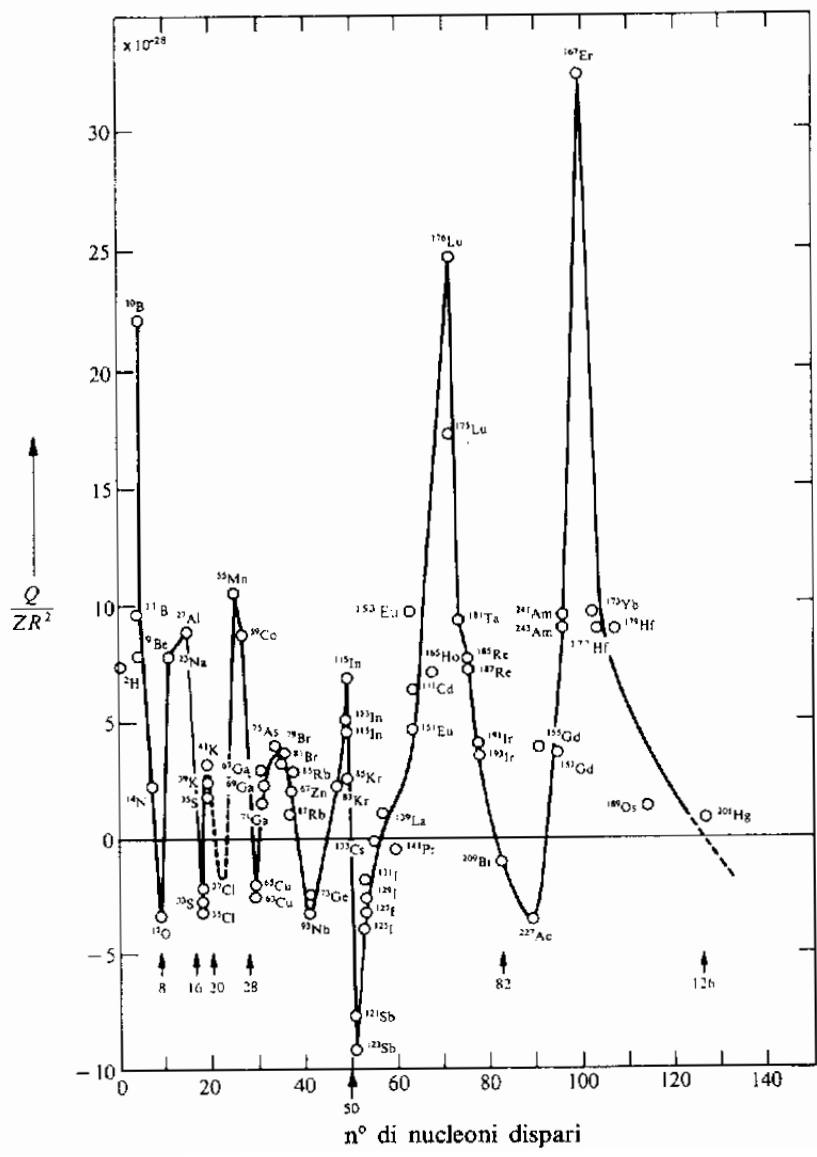
Figura 4: Momenti nucleari ridotti di quadrupolo elettrico, in funzione del numero d'ordine del nucleone dispari. La quantità Q/ZR^2 fornisce una misura della deformazione nucleare indipendente dalla grandezza del nucleo.
