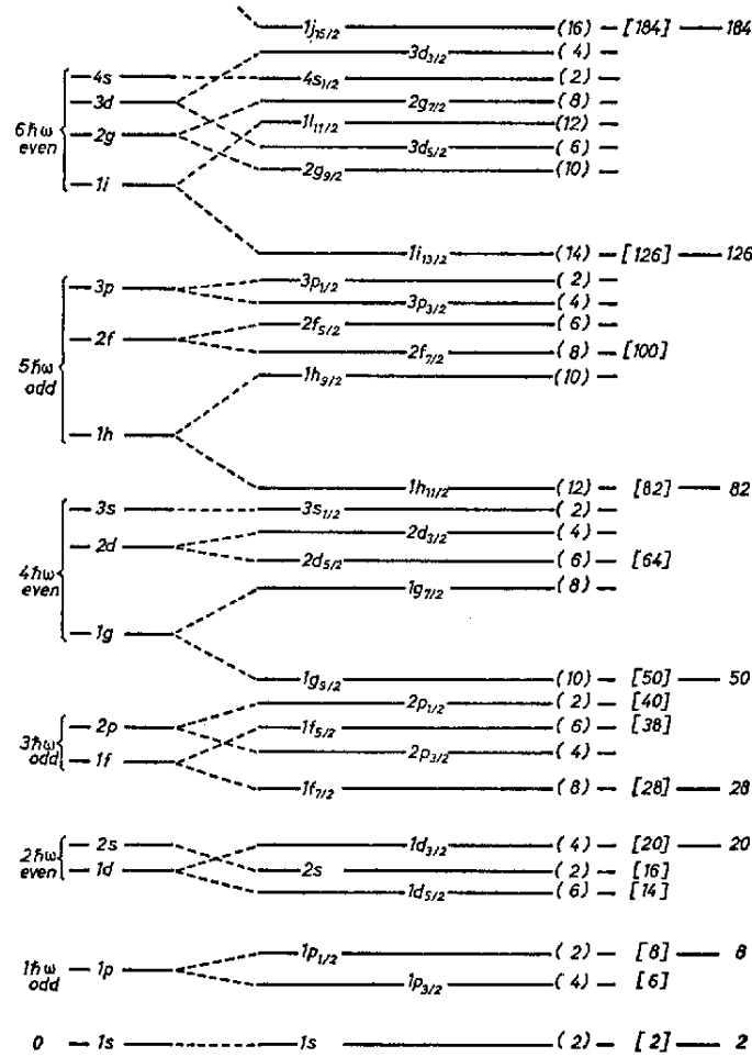
Figura 9: Schema dei livelli di singola particella per un potenziale centrale intermedio tra oscillatore armonico e buca a pareti infinite, con in aggiunta un termine di spin-orbita. I numeri di nucleoni occupanti ogni singolo livello sono indicati tra parentesi tonde. Il numero cumulativo tra parentesi quadre.
