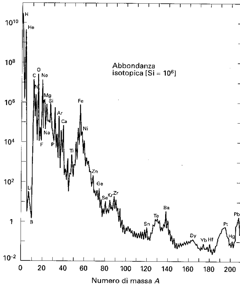
Figura 3: Abbondanza degli elementi del sistema solare in funzione del numero di massa A, normalizzata all'abbondanza del silicio (=10 6 ).
