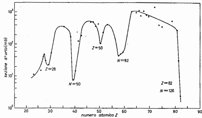
Figura 6: Sezione d'urto di cattura neutronica, per neutroni di energia di 30 keV, in funzione del numero di protoni.
