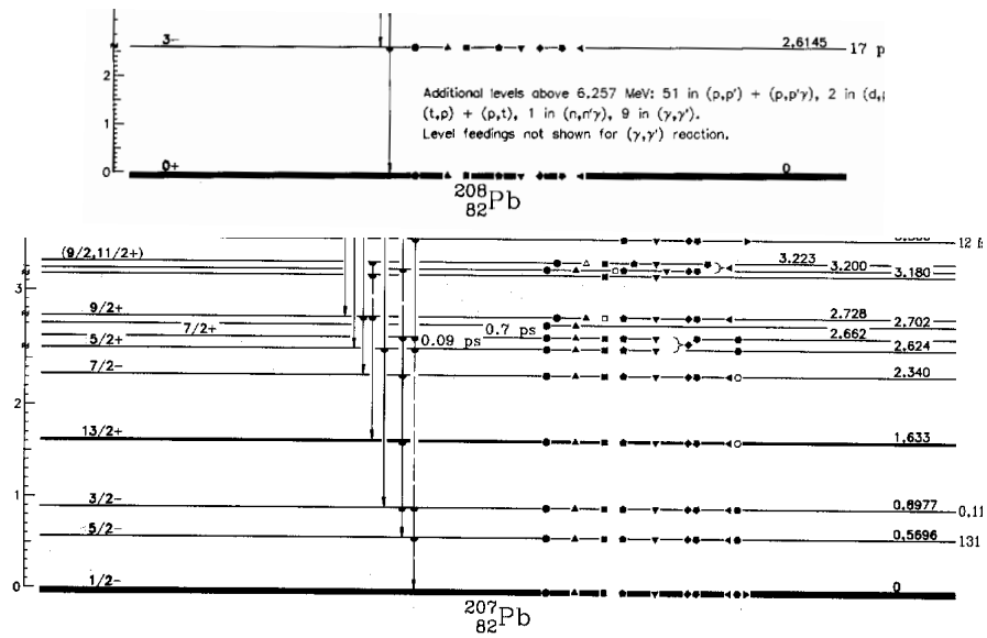
Figura 5: Schema dei livelli del ^{208}\text{Pb} , doppio magico, e del ^{207}\text{Pb} semi-magico, per energie di eccitazione fino a 3 MeV.
