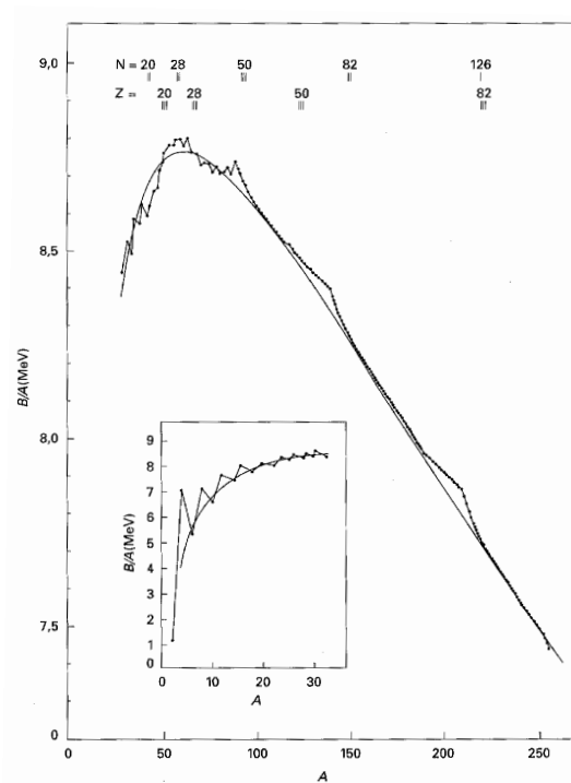
Figura 2: Energia di legame per nucleone nei nuclei con numero di massa A pari. La linea continua corrisponde alla formula semi-empirica della massa di Weißäcker. Nel riquadro sono presentate le energie di legame di nuclei leggeri. Anche nei nuclei più pesanti si possono osservare delle deviazioni in corrispondenza ai numeri magici. I nuclei magici sono più legati degli altri.
