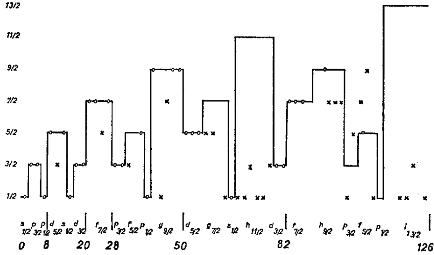
Figura 10: Spin di nuclei con numero dispari di neutroni. La linea presenta le previsioni del modello a shell, cerchi e crocette sono i rappresentano i valori empirici.
