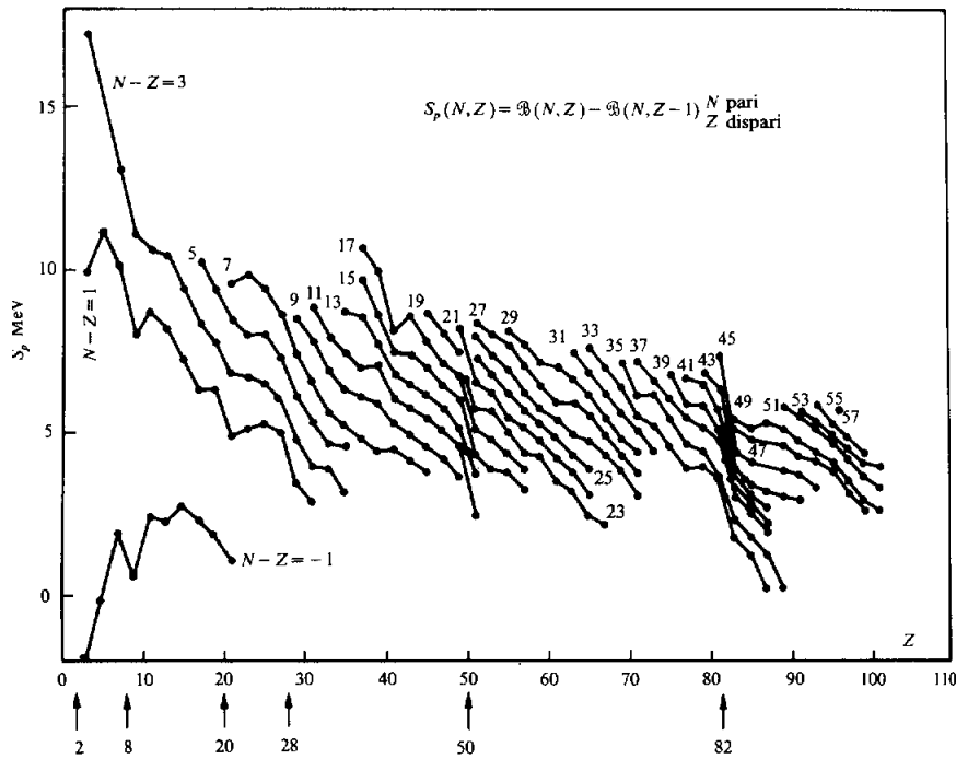
Figura 7: Energie di separazione dei neutroni.
