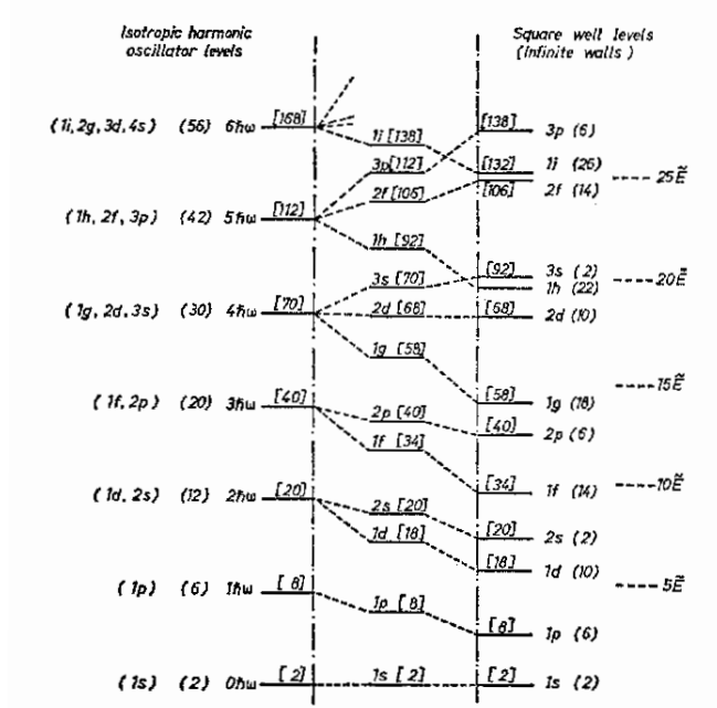
Figura 8: Schema dei livelli si singola particella per tre potenziali centrali, oscillatore armonico, buca quadrata e un potenziale intermedio.
