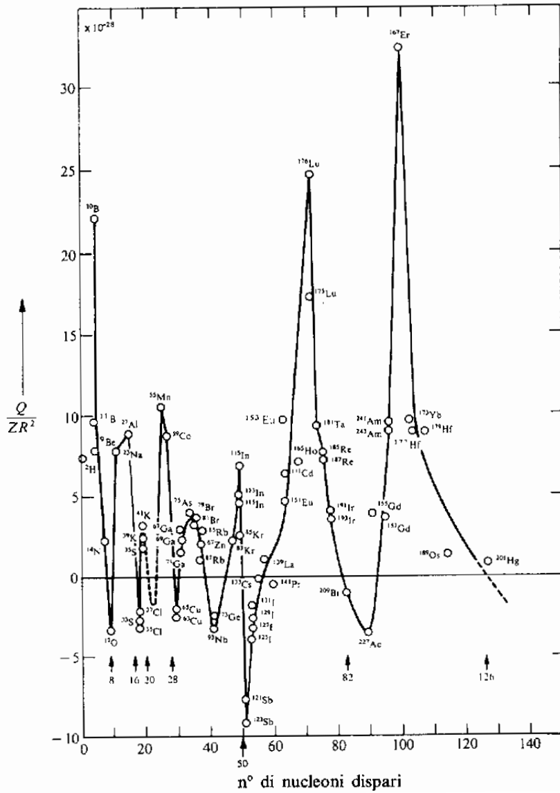
Figura 1.4: Momenti nucleari ridotti di quadrupolo elettrico, in funzione del numero d'ordine del nucleone dispari. La quantità Q/ZR^2 fornisce una misura della deformazione nucleare indipendente dalla grandezza del nucleo.
