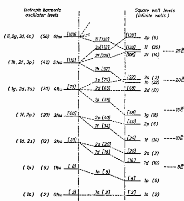
Figura 1.8: Schema dei livelli di singola particella per tre potenziali centrali, oscillatore armonico, buca quadrata e un potenziale intermedio.
