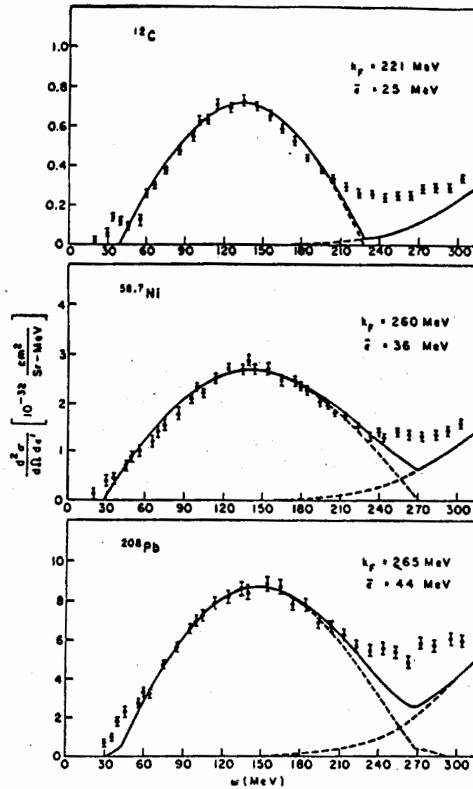
Figura 1.1: Sezioni d'urto di diffusione anelastica di elettroni su nuclei nella regione del picco quasi-elastico, calcolate con il modello a gas di Fermi e confrontate con dati sperimentali.
