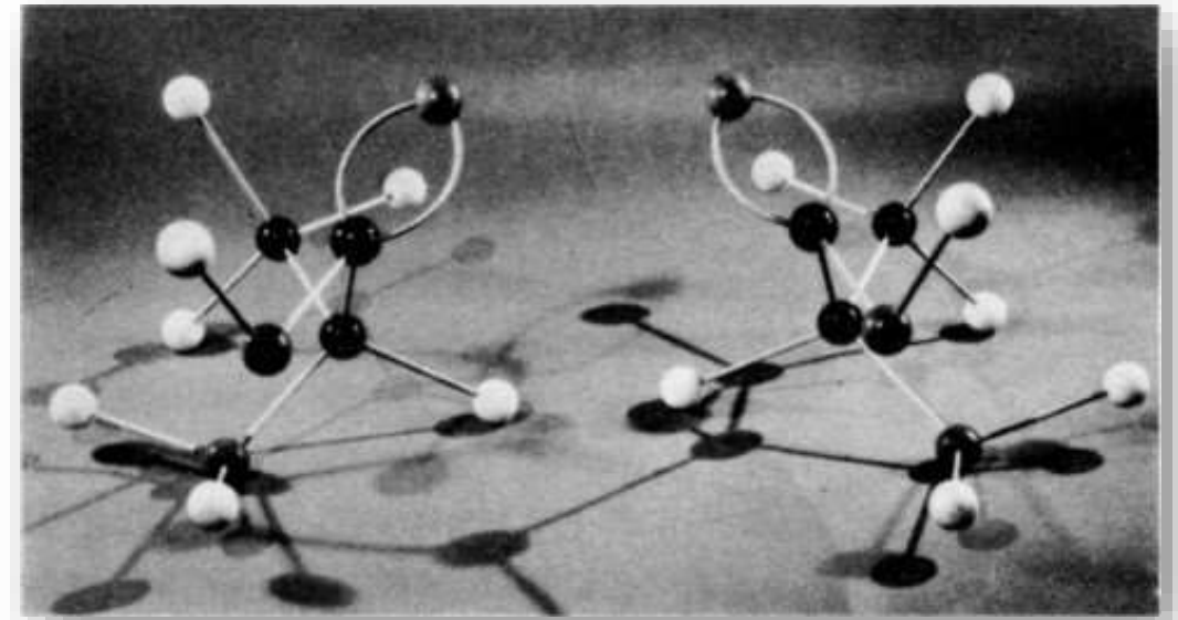
L-alanina (a)
