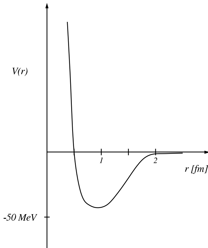
Figura 1.3: Potenziale nucleone-nucleone nel canale scalare.
