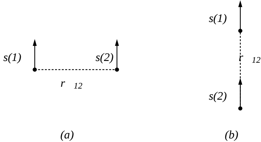
Figura 1.2: Geometrie in cui il termine tensoriale del potenziale nucleone-nucleone agisce in maniera differente.
