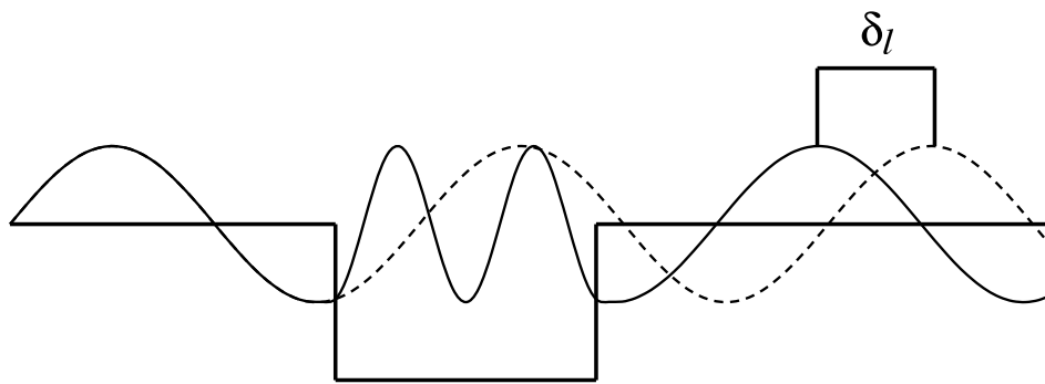
Figura 1.1: Schematizzazione del processo di diffusione da potenziale. La linea tratteggiata rappresenta la soluzione senza potenziale, mentre la linea continua quella in presenza di un potenziale attivo in una regione limitata dello spazio. Asintoticamente le due soluzioni differiscono solo per uno sfasamento.
