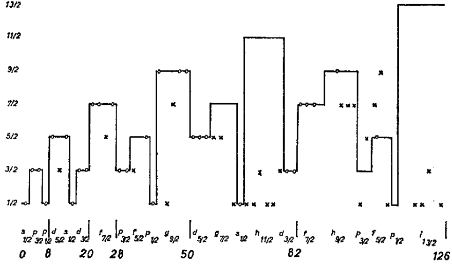
Figura 1.10: Spin di nuclei con numero dispari di neutroni. La linea presenta le previsioni del modello a shell, cerchi e crocette sono i rappresentano i valori empirici.
