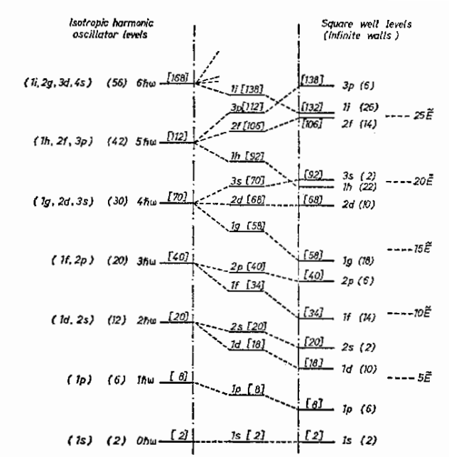
Figura 1.8: Schema dei livelli si singola particella per tre potenziali centrali, oscillatore armonico, buca quadrata e un potenziale intermedio.
