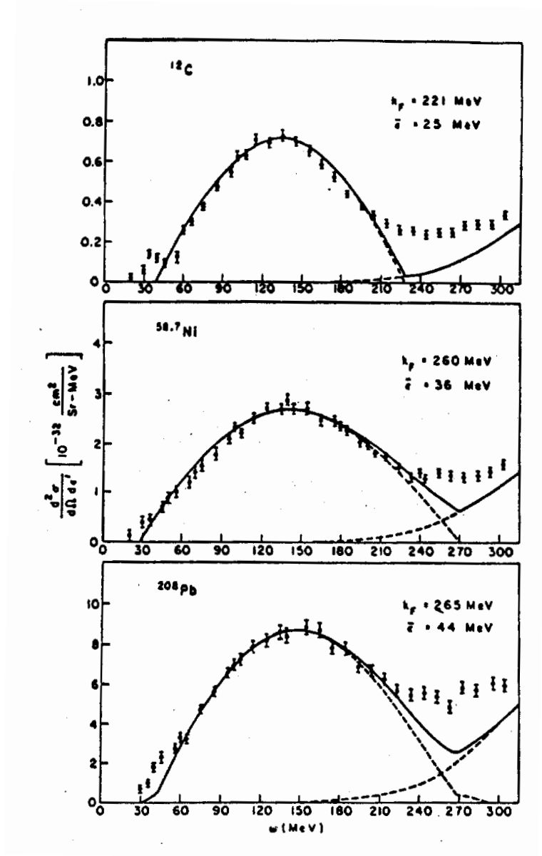
Figura 1.1: Sezioni d'urto di diffusione anelastica di elettroni su nuclei nella regione del picco quasi-elastico, calcolate con il modello a gas di Fermi e confrontate con dati sperimentali.
