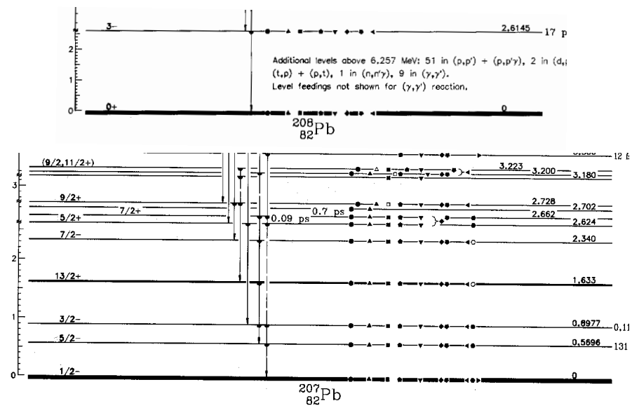
Figura 1.5: Schema dei livelli del ^{208}\text{Pb} , doppio magico, e del ^{207}\text{Pb} semi-magico, per energie di eccitazione fino a 3 MeV.
