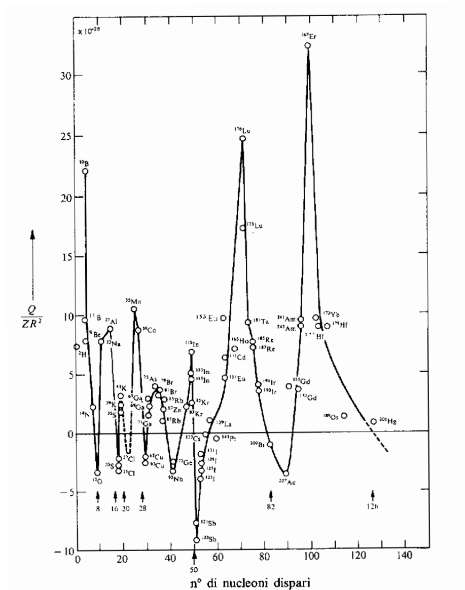
Figura 1.4: Momenti nucleari ridotti di quadrupolo elettrico, in funzione del numero d'ordine del nucleone dispari. La quantità Q/ZR^2 fornisce una misura della deformazione nucleare indipendente dalla grandezza del nucleo.
