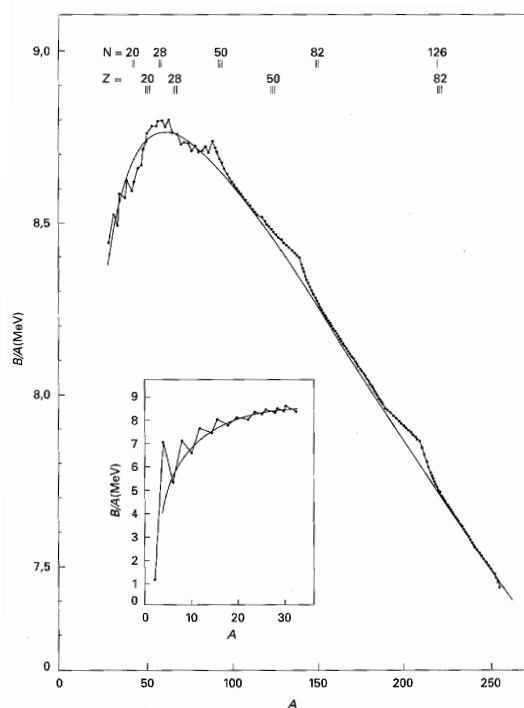
Figura 1.2: Energia di legame per nucleone nei nuclei con numero di massa A pari. La linea continua corrisponde alla formula semi-empirica della massa di Weizsäcker. Nel riquadro sono presentate le energie di legame di nuclei leggeri. Anche nei nuclei più pesanti si possono osservare delle deviazioni in corrispondenza ai numeri magici. I nuclei magici sono più legati degli altri.
