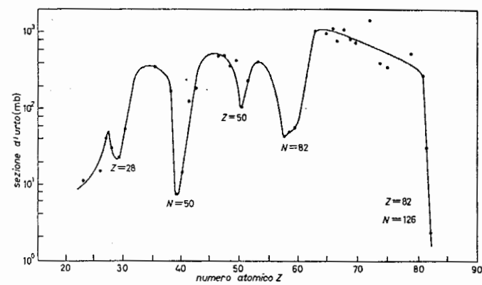
Figura 1.6: Sezione d’urto di cattura neutronica, per neutroni di energia di 30 keV, in funzione del numero di protoni.
