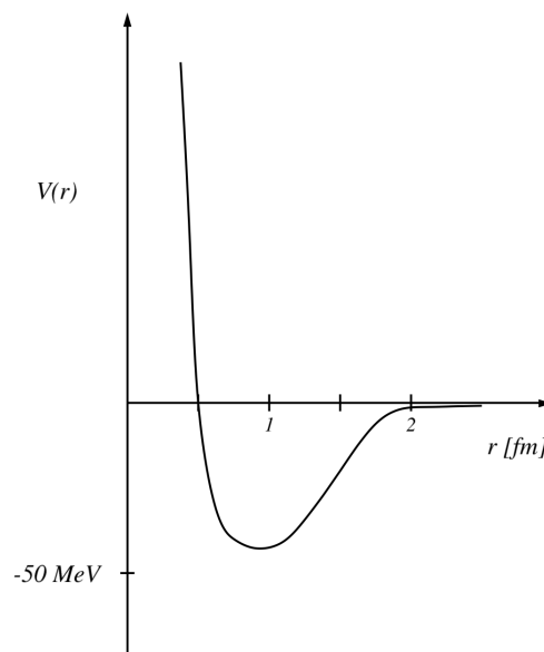
Figura 12: Schema della parte scalare dell'interazione tra due nucleoni.
