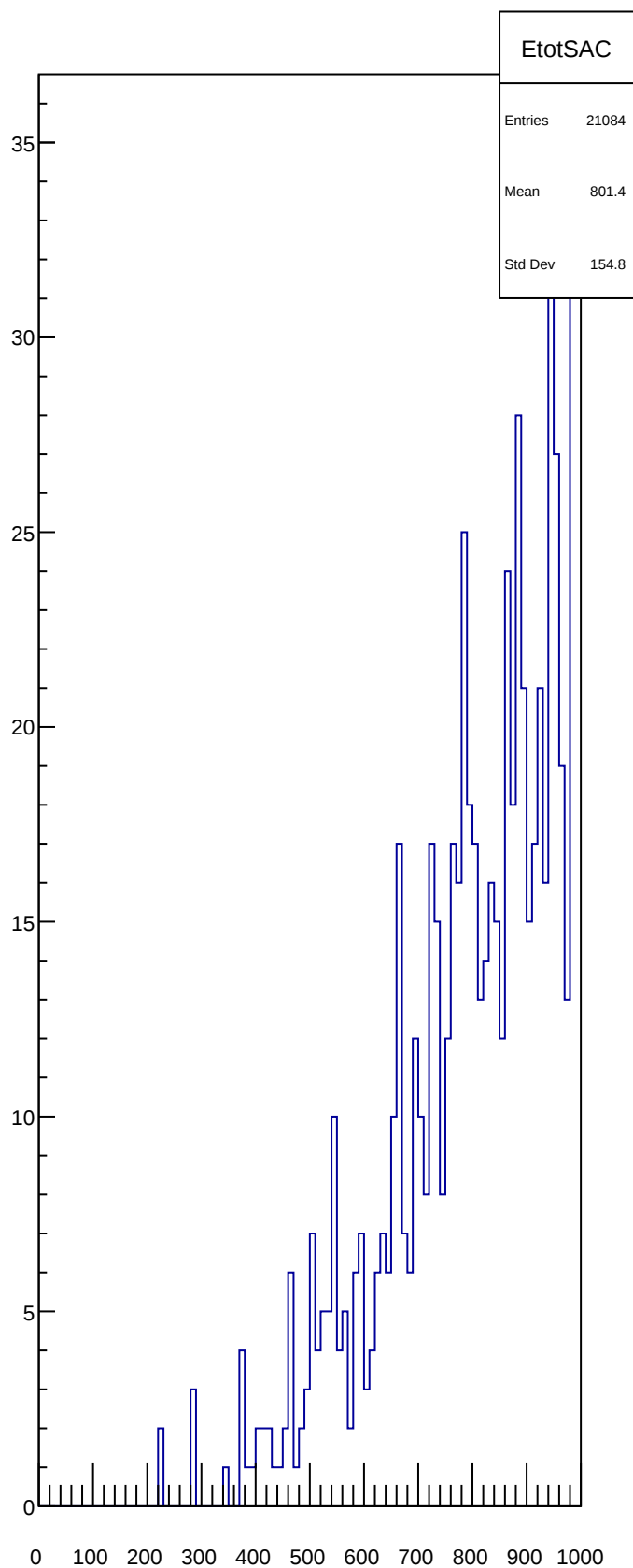
EtotSAC
