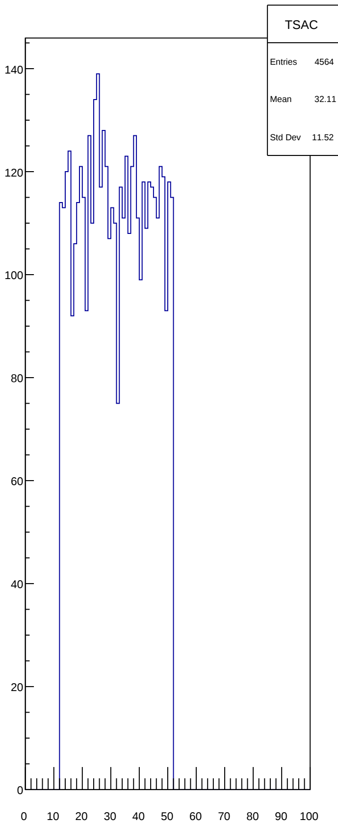
TSAC
