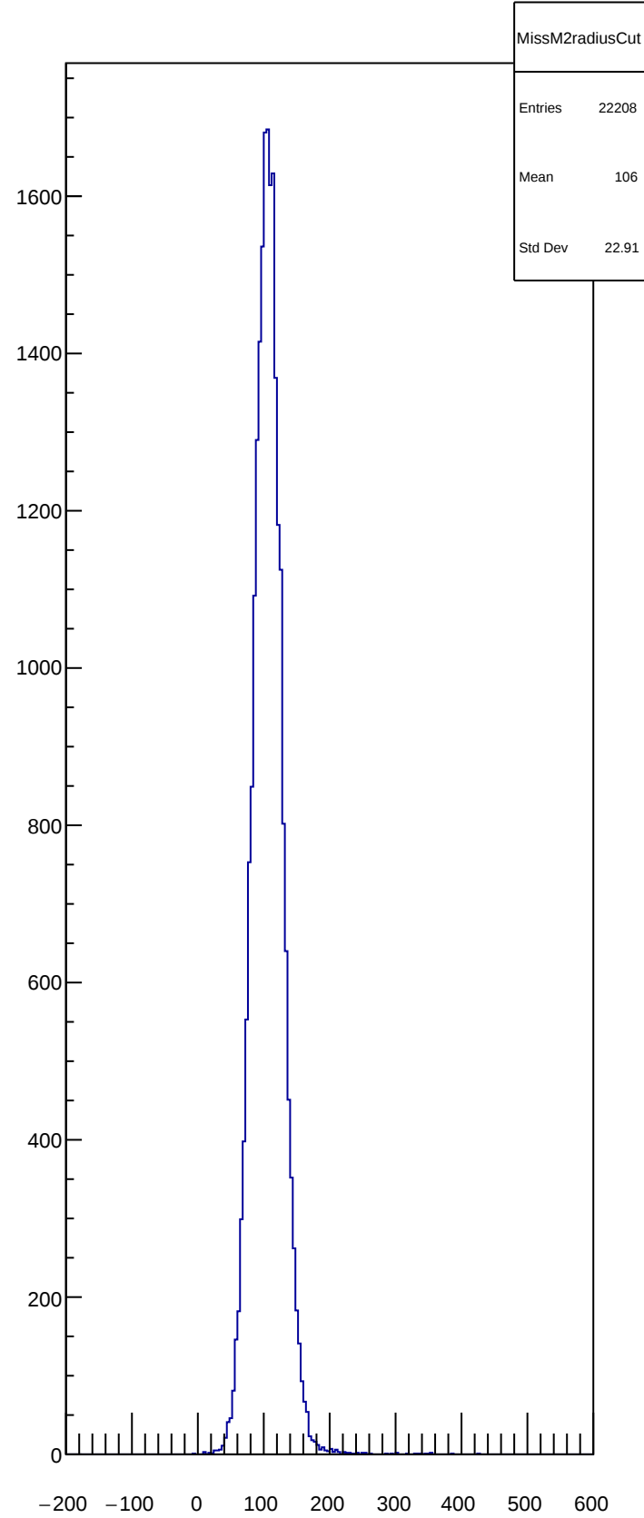
MissM2radiusCut
