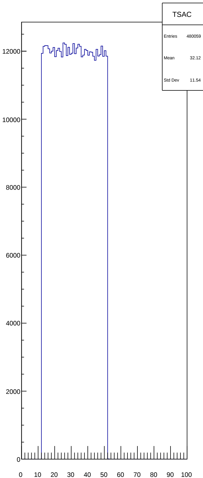
TSAC
