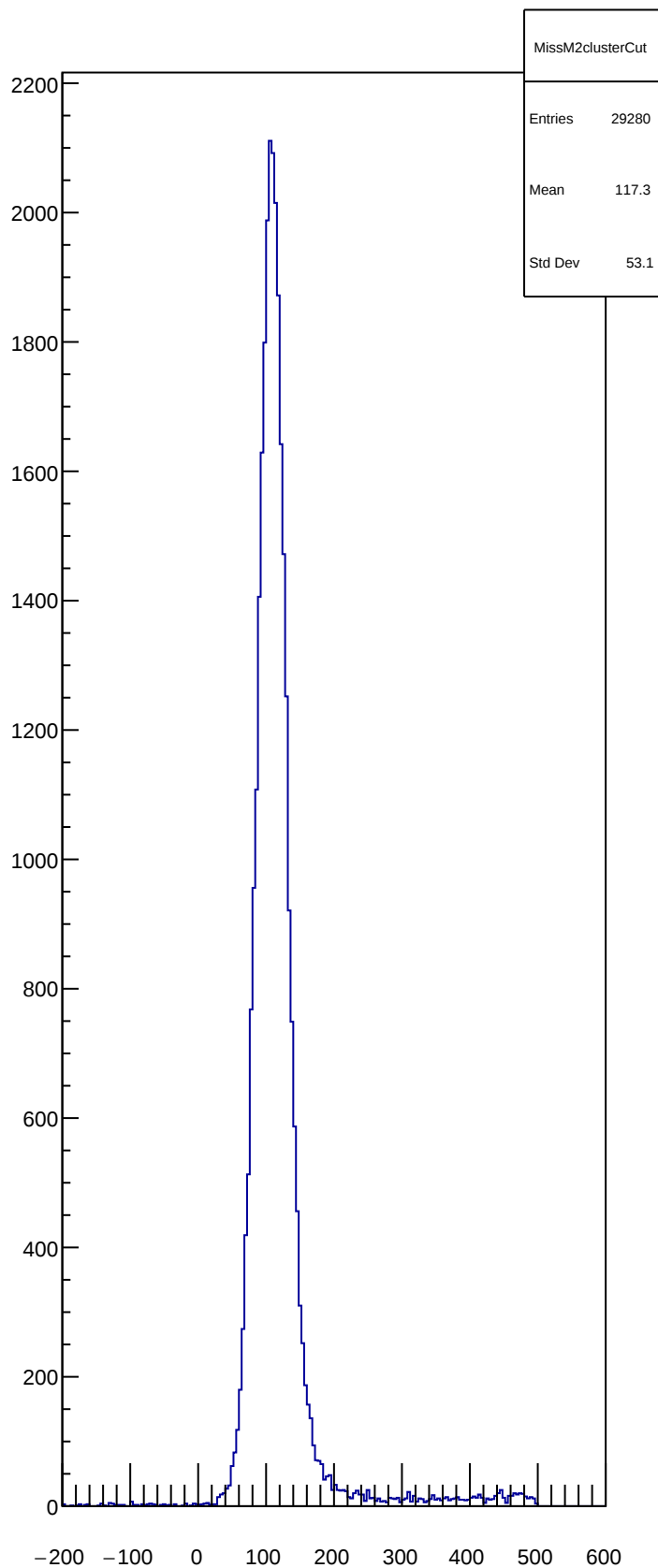
MissM2clusterCut
