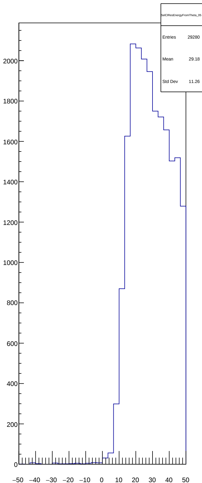
SelClResEnergyFromTheta_05
