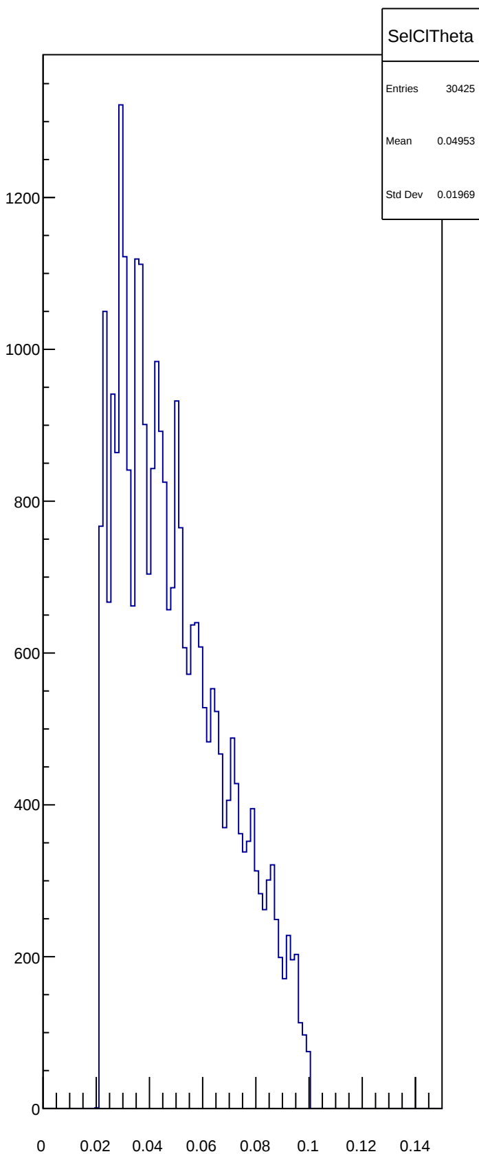
SelCITheta
