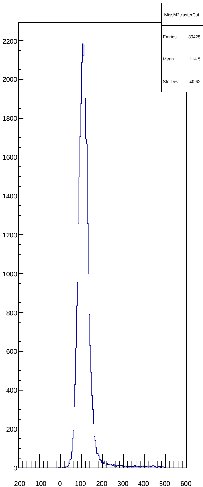
MissM2clusterCut
