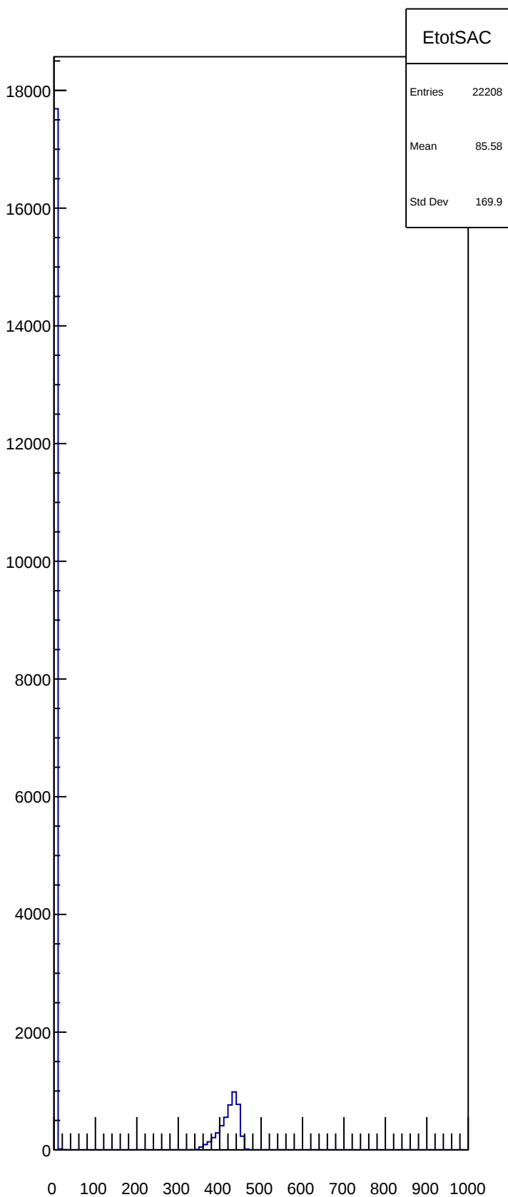
EtotSAC
