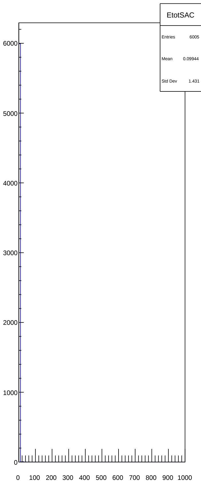
EtotSAC
