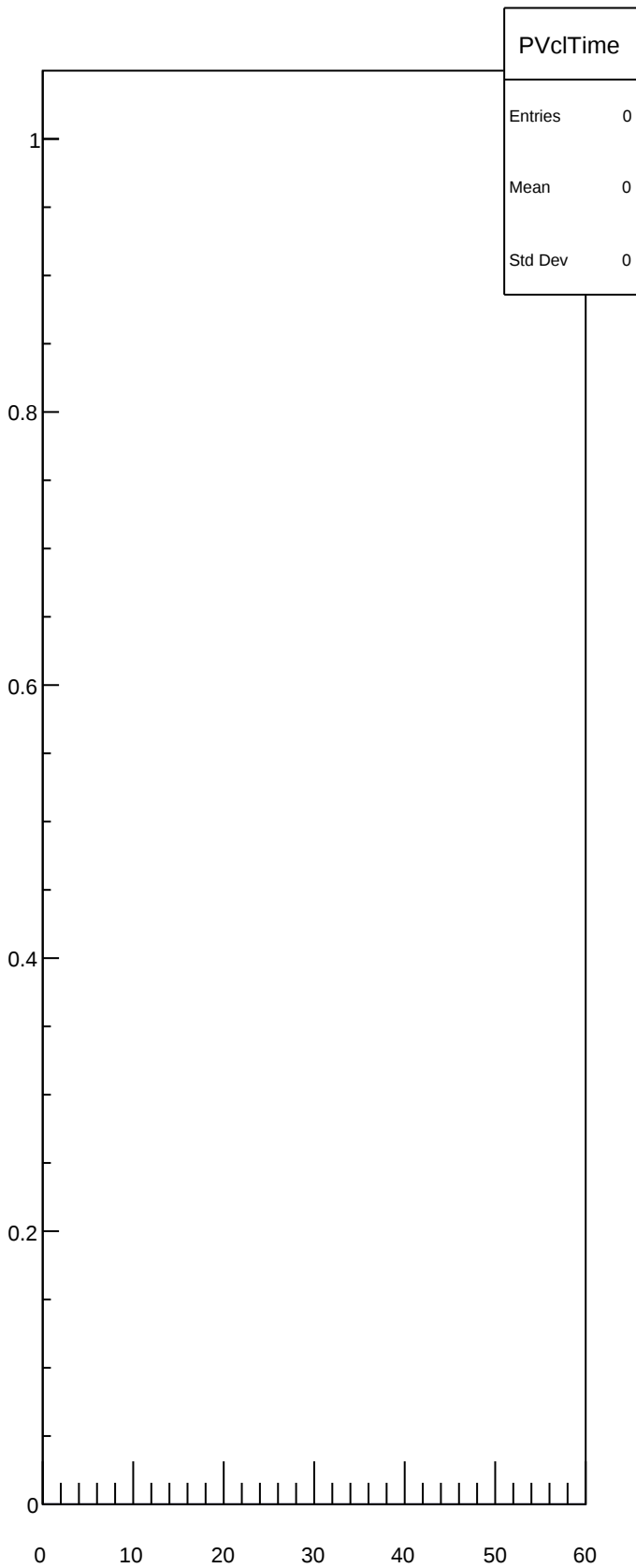
PVclTime
