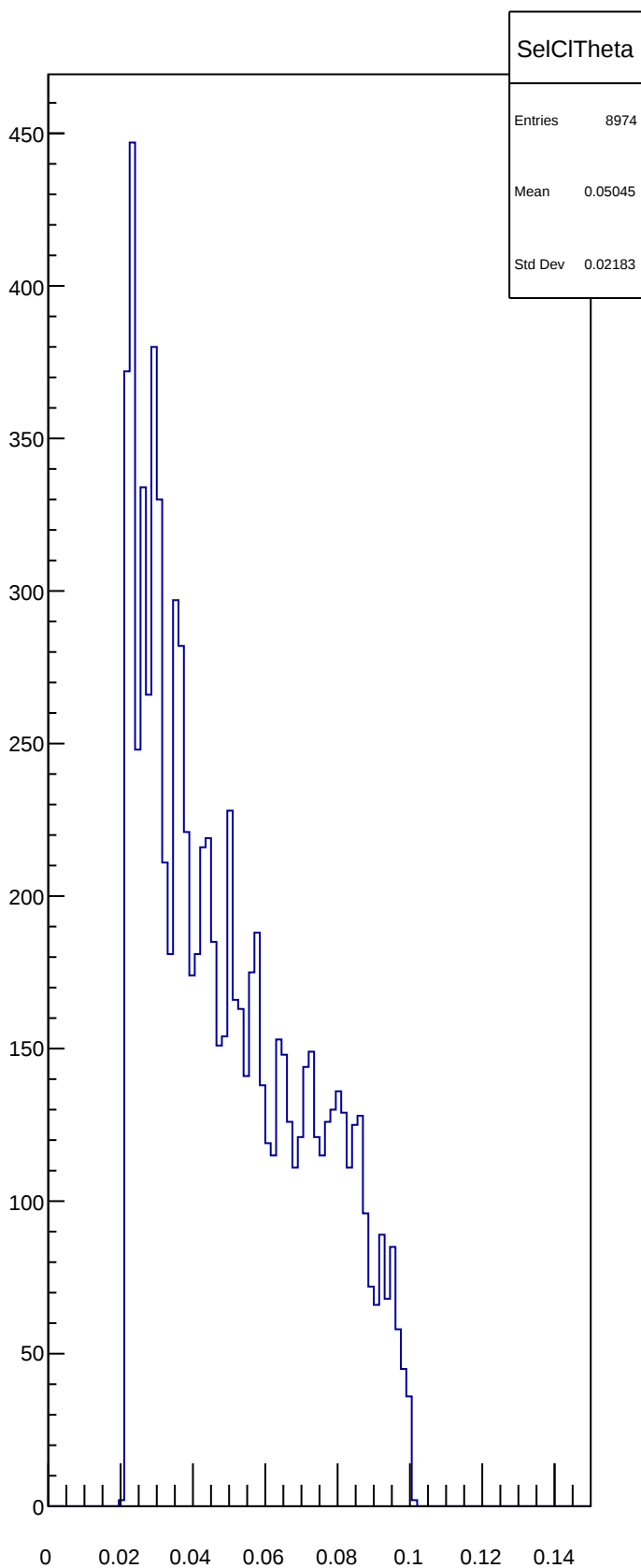
SelCITheta
