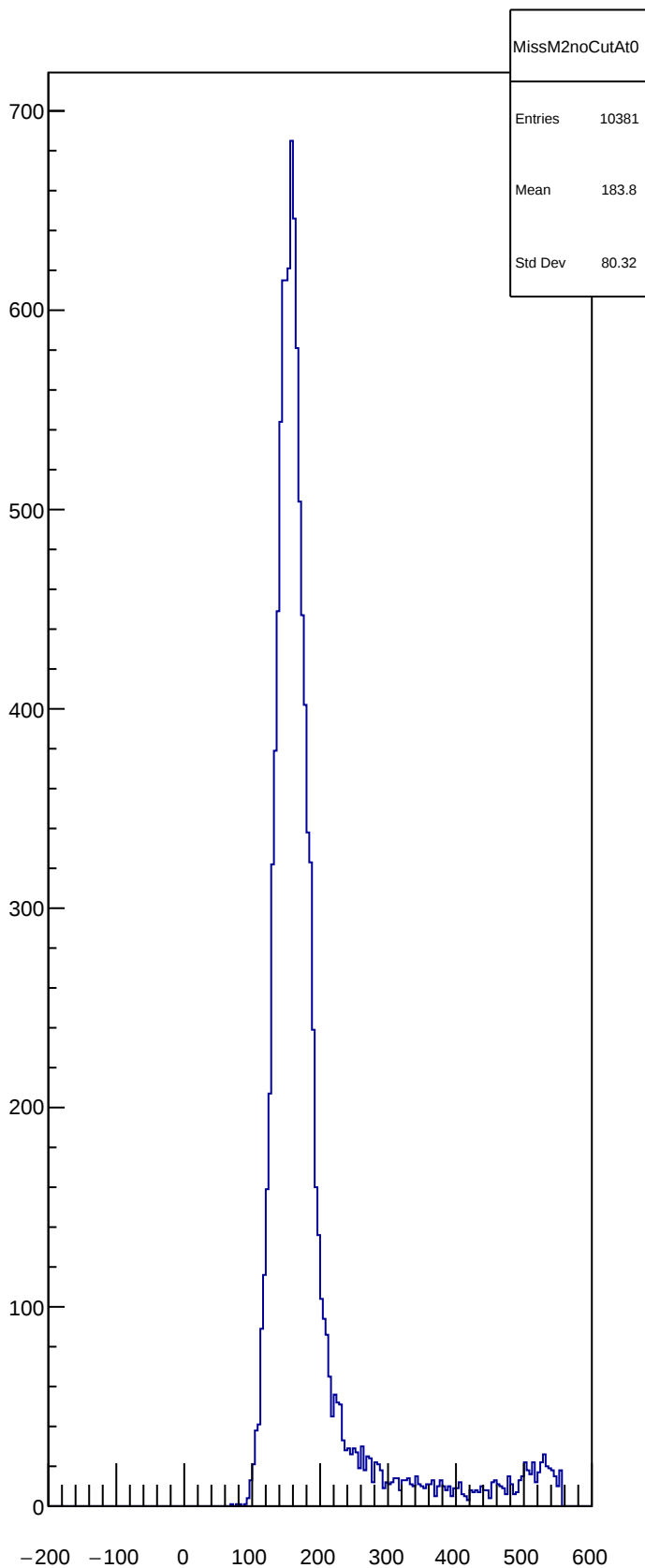
MissM2noCutAt0
