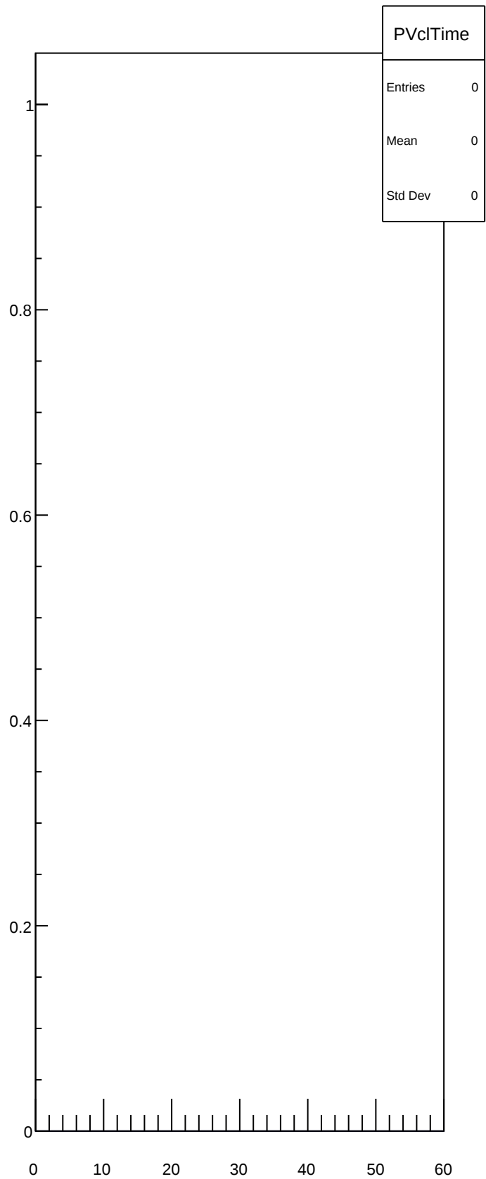
PVclTime
