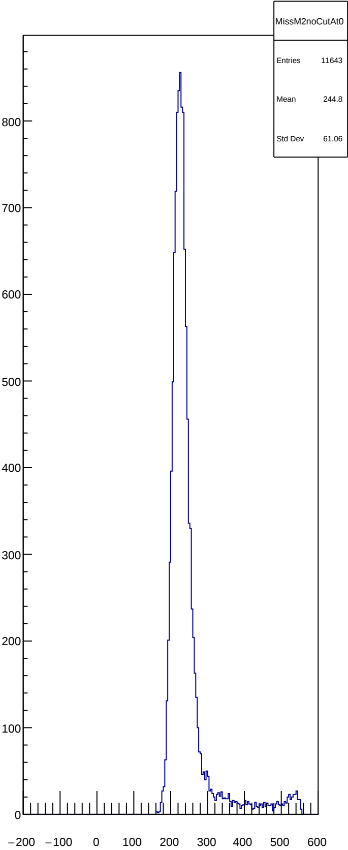
MissM2noCutAt0
