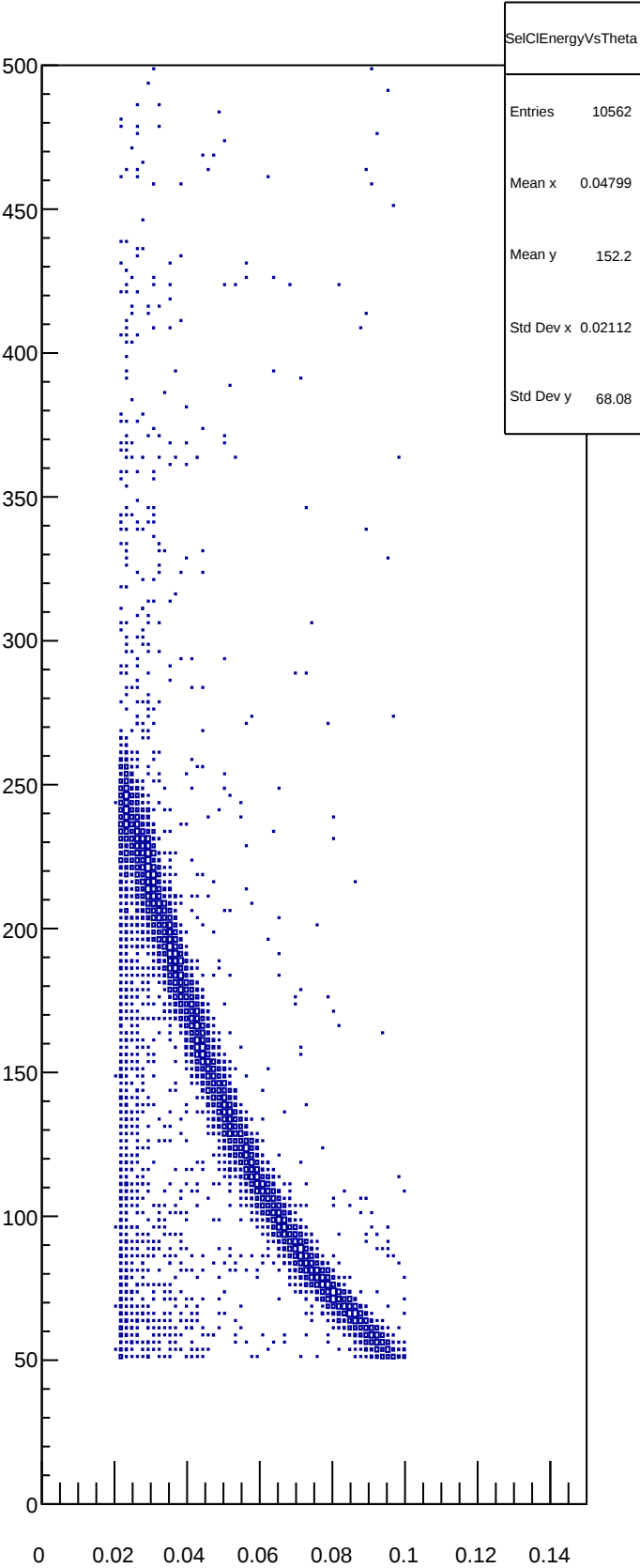
SelCIEnergyVsTheta
