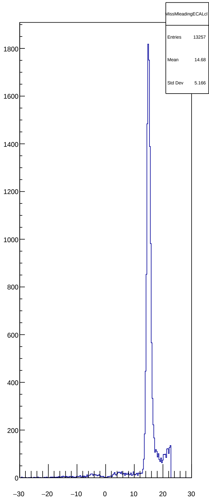
MissMleadingECALcl
