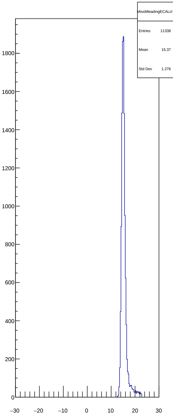
MissMleadingECALcl
