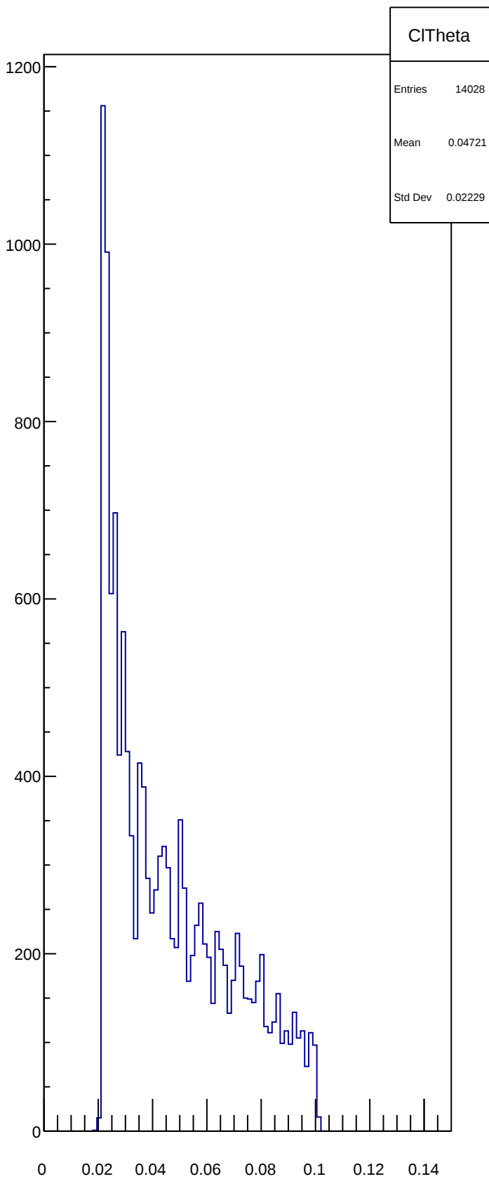
CITheta
