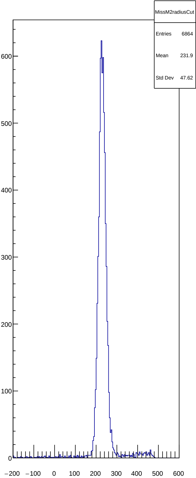
MissM2radiusCut
