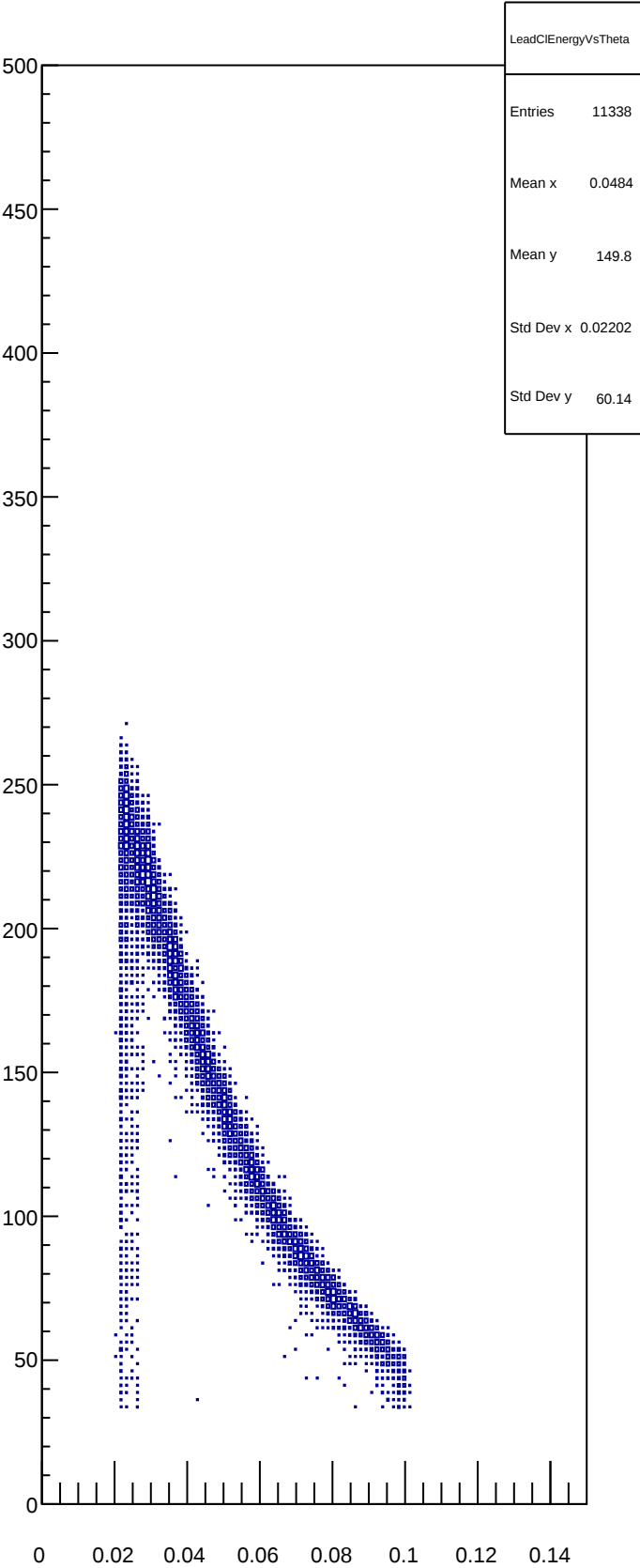
LeadClEnergyVsTheta
