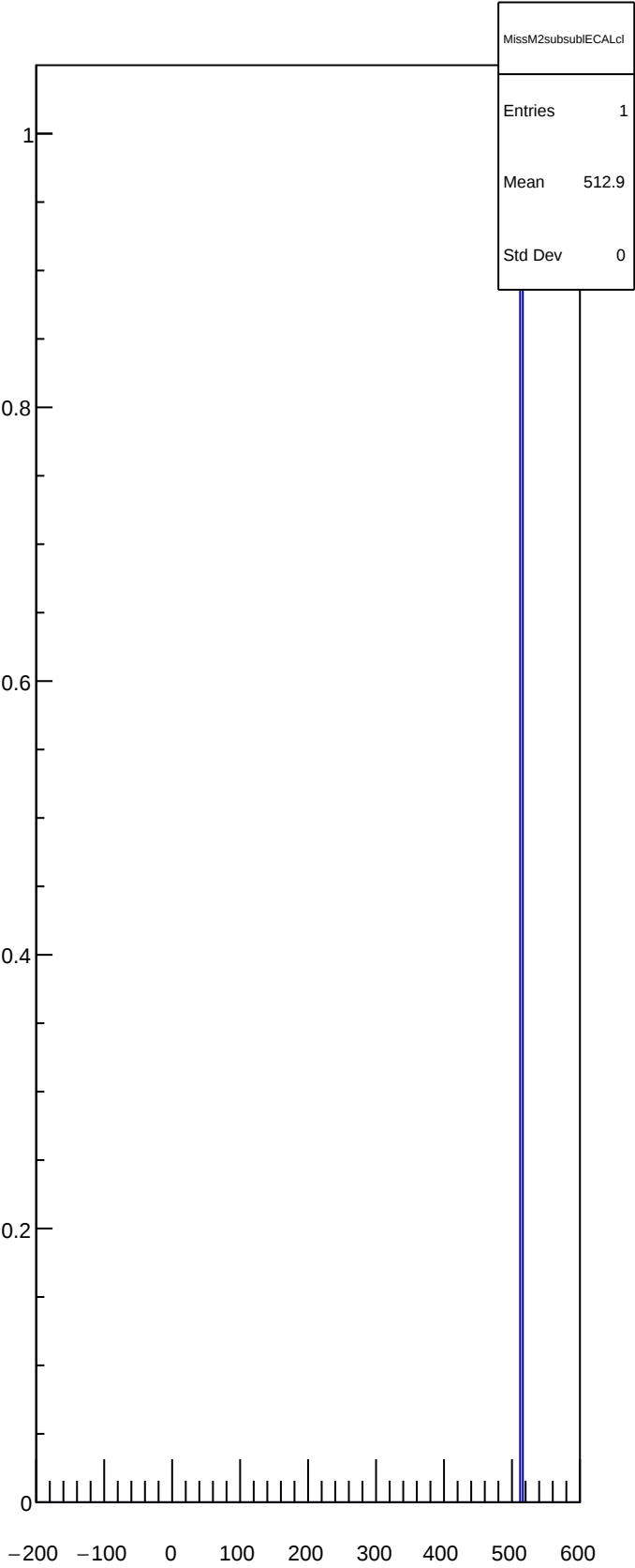
MissM2subsubIECALcl
