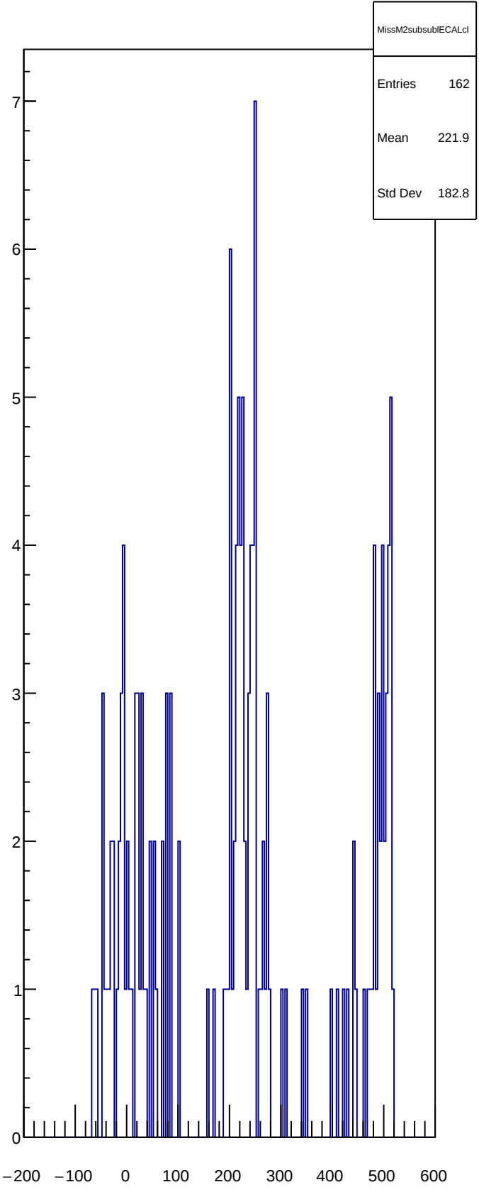
MissM2subsubIECALcl
