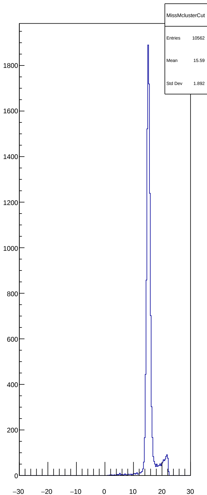
MissMclusterCut
