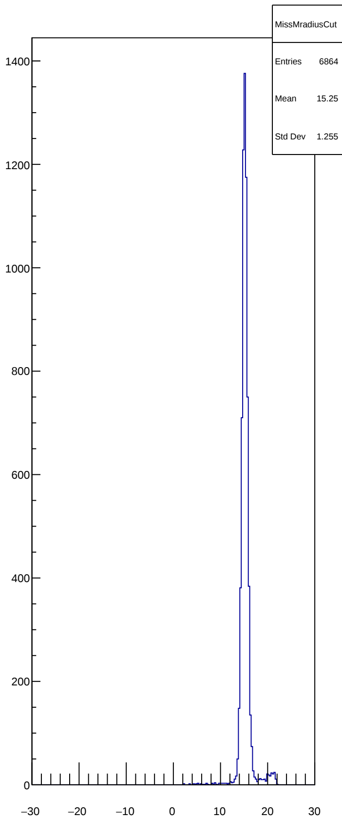
MissMradiusCut
