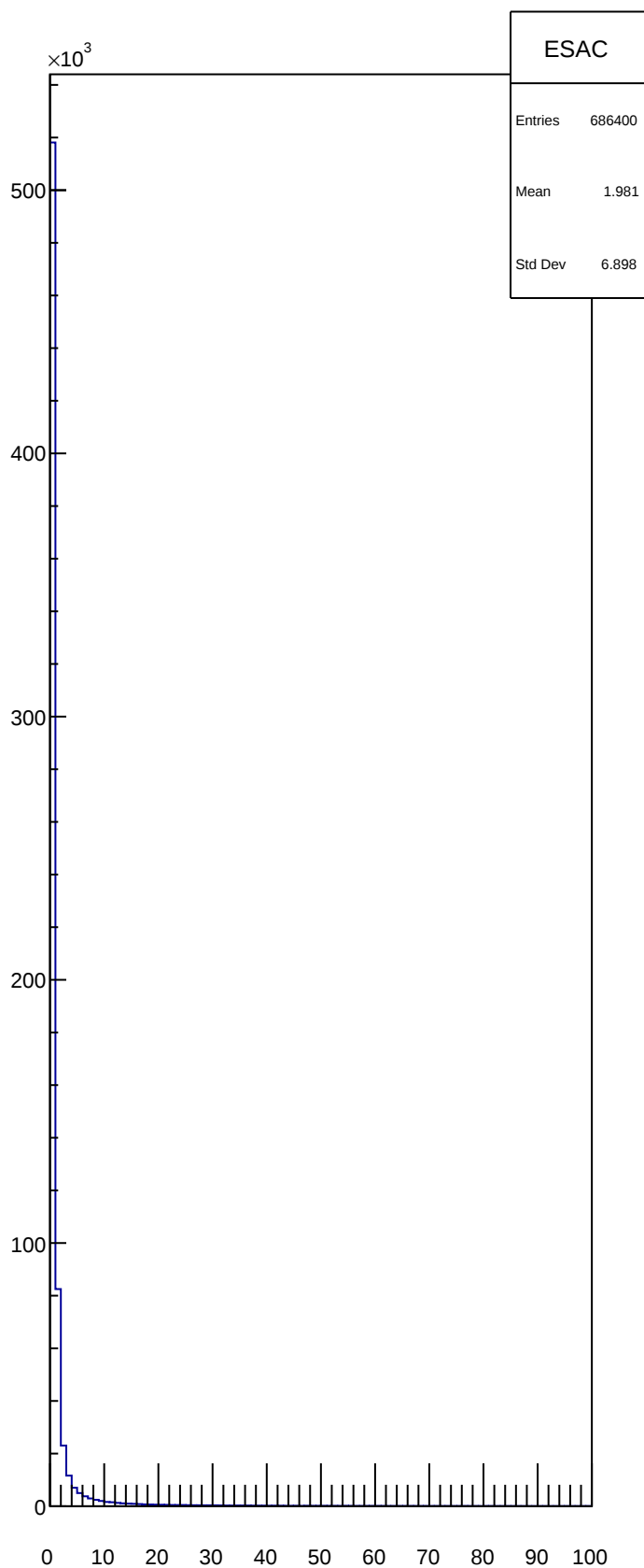
ESAC
