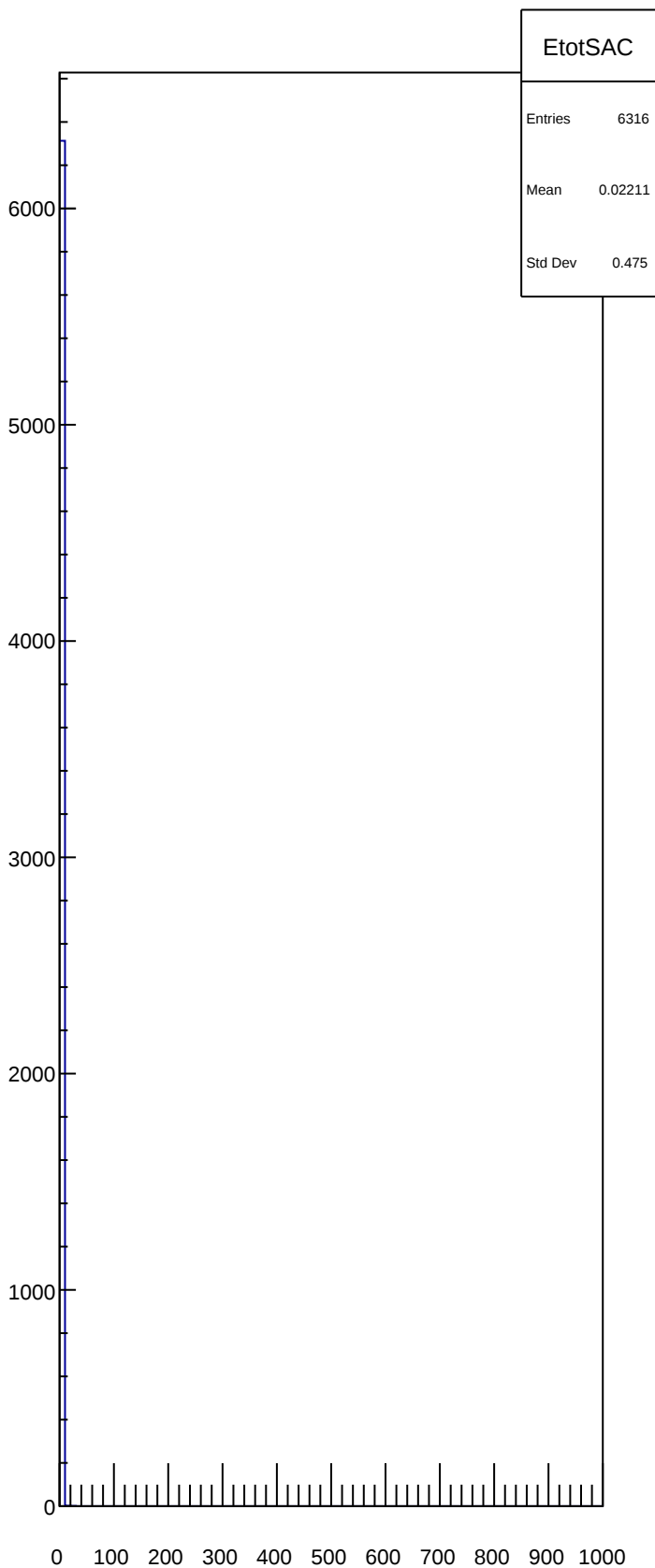
EtotSAC
