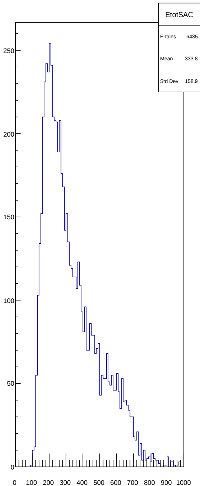
EtotSAC
