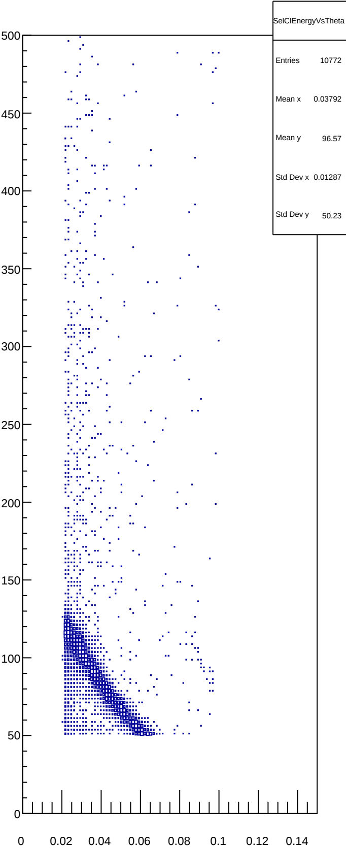
SelClEnergyVsTheta
