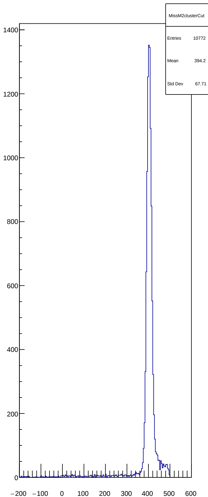
MissM2clusterCut
