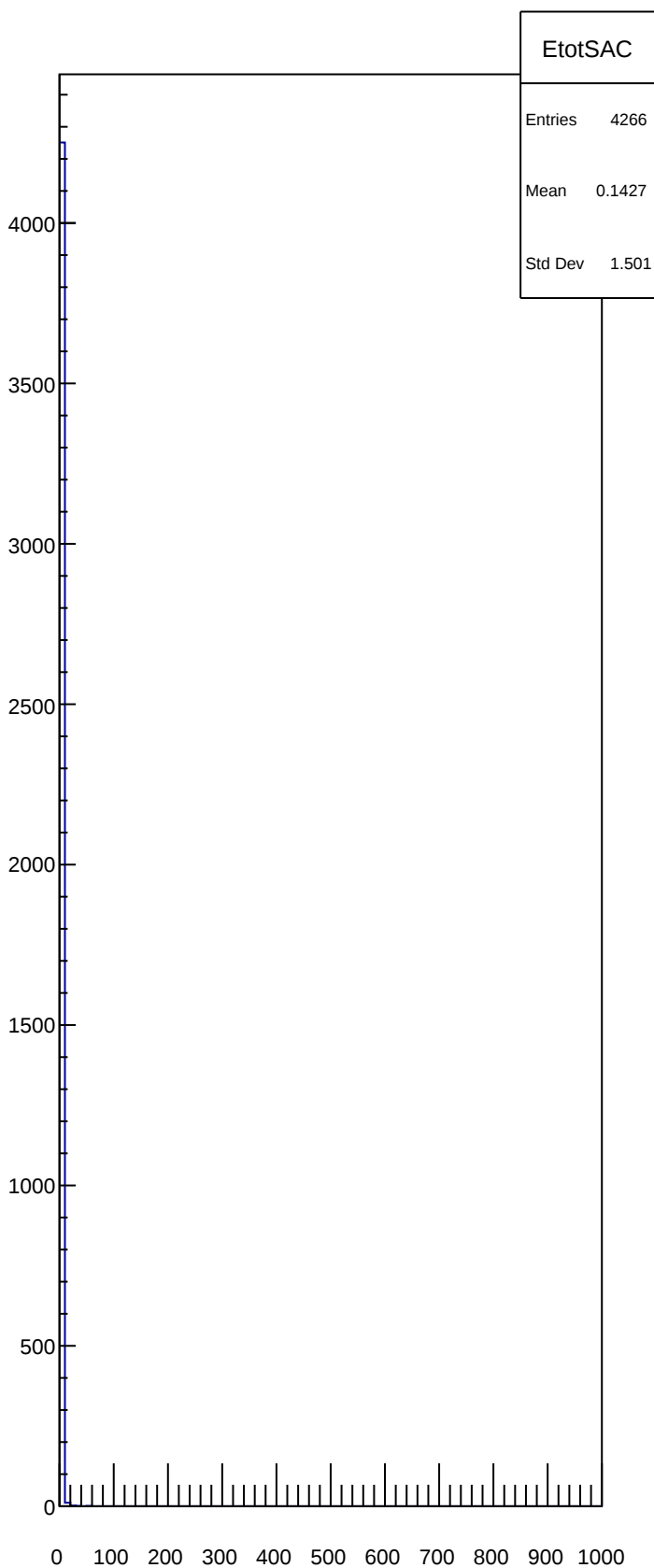
EtotSAC
