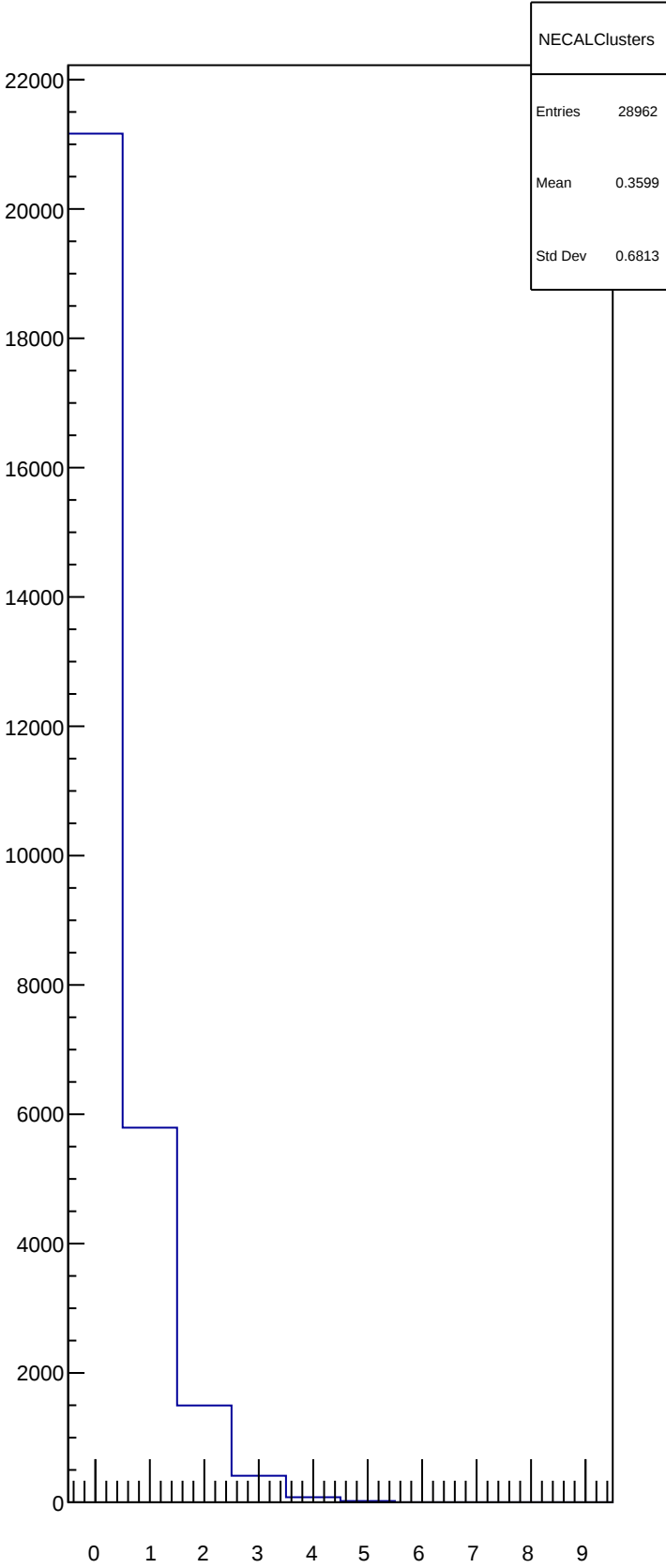
NECALClusters
