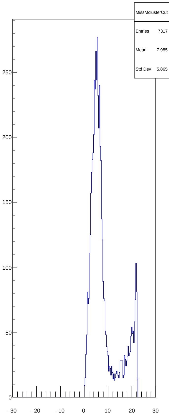
MissMclusterCut
