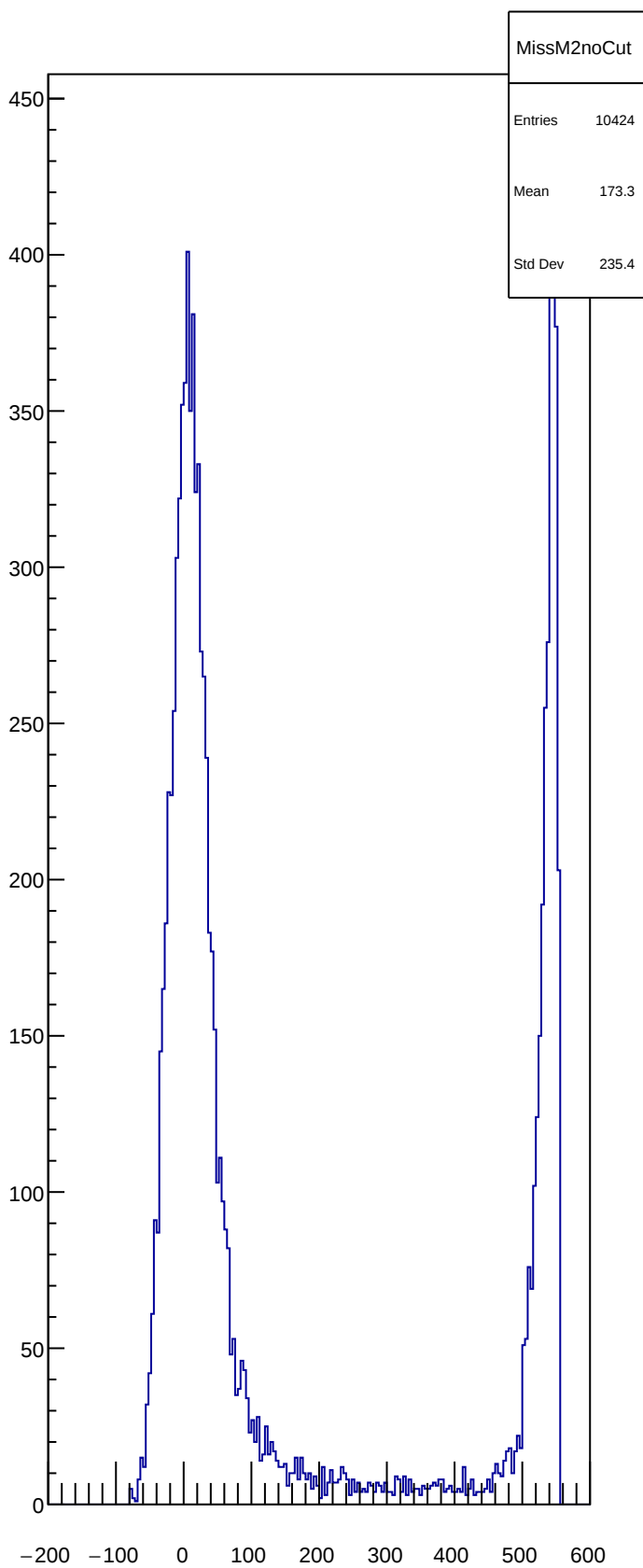
MissM2noCut
