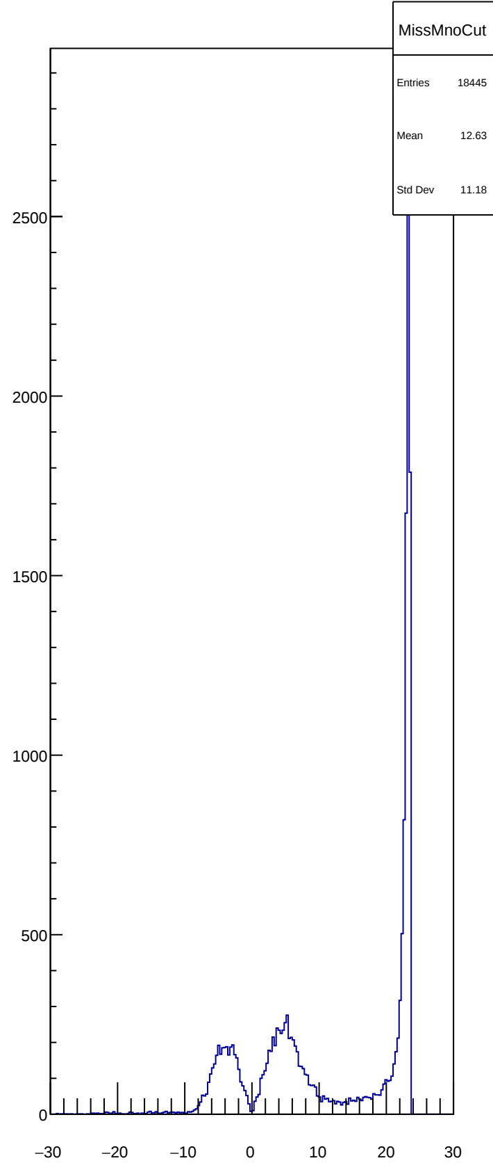
MissMnoCut
