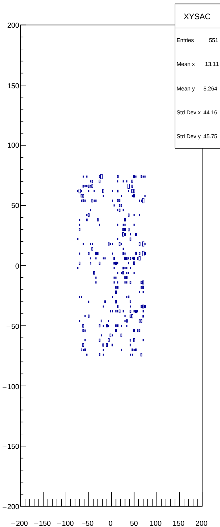
XY SAC
