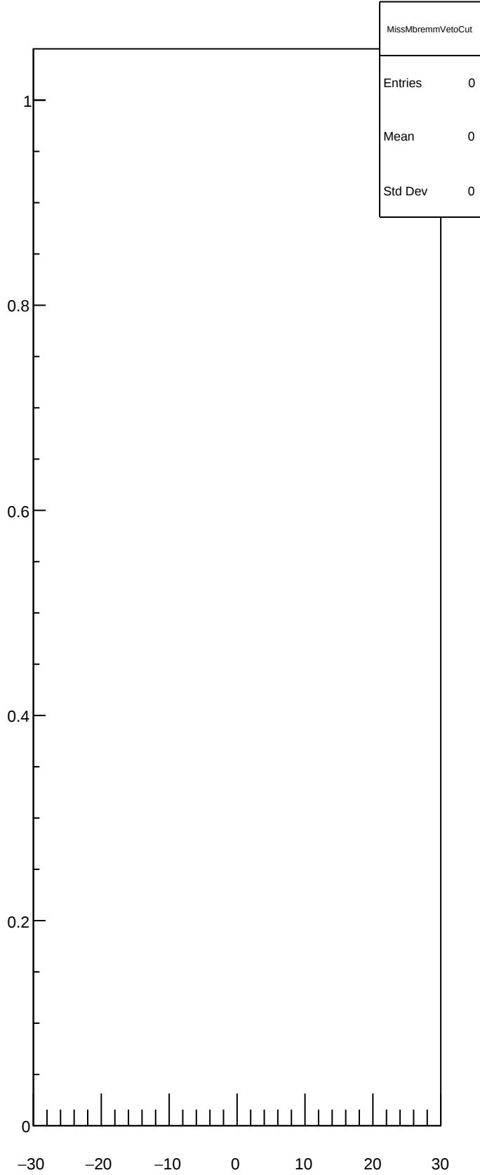
MissMbremmVetoCut
