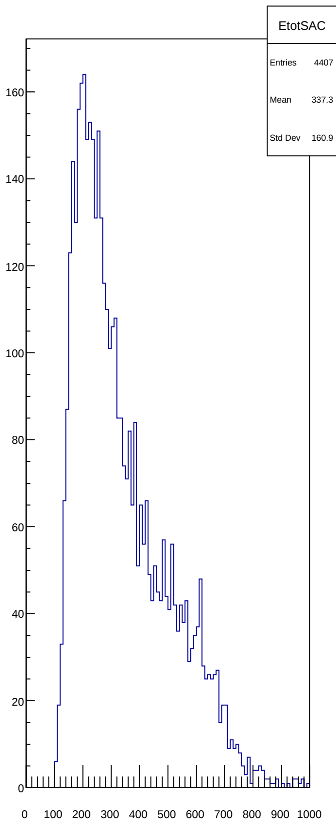
EtotSAC
