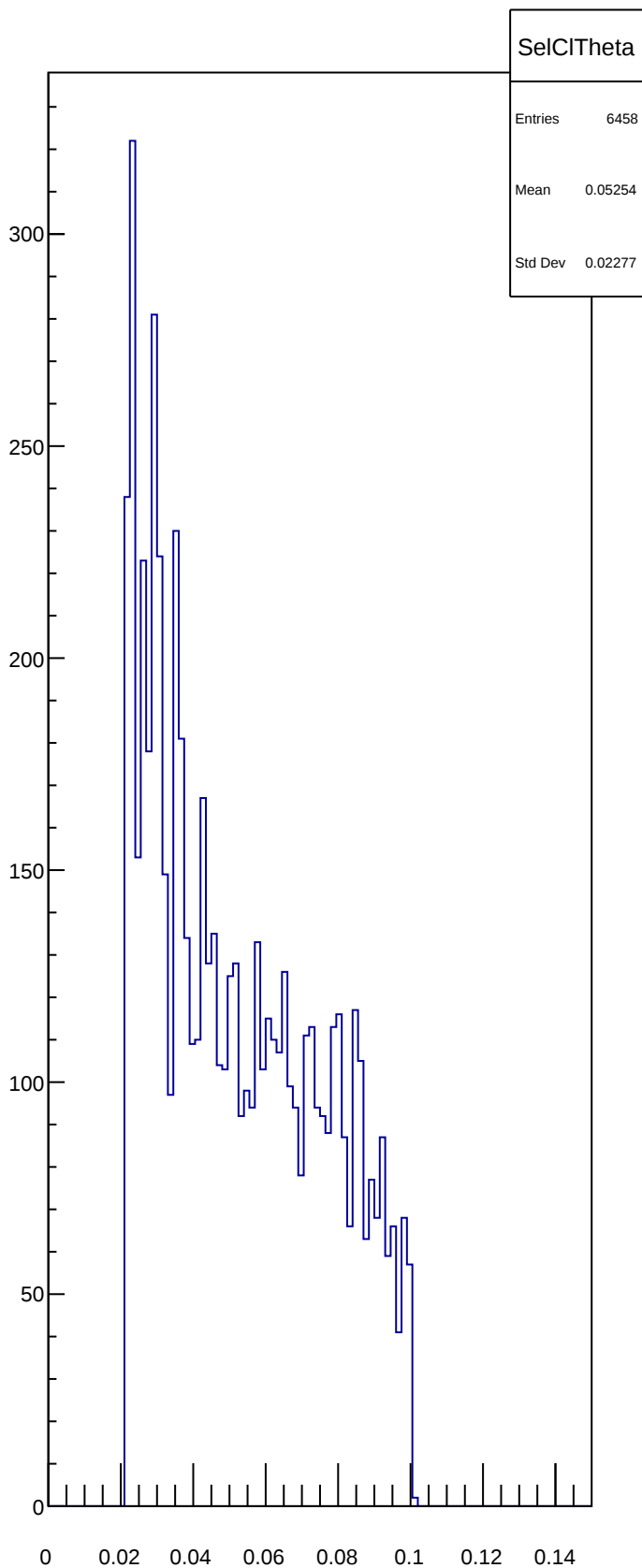
SelCITheta
