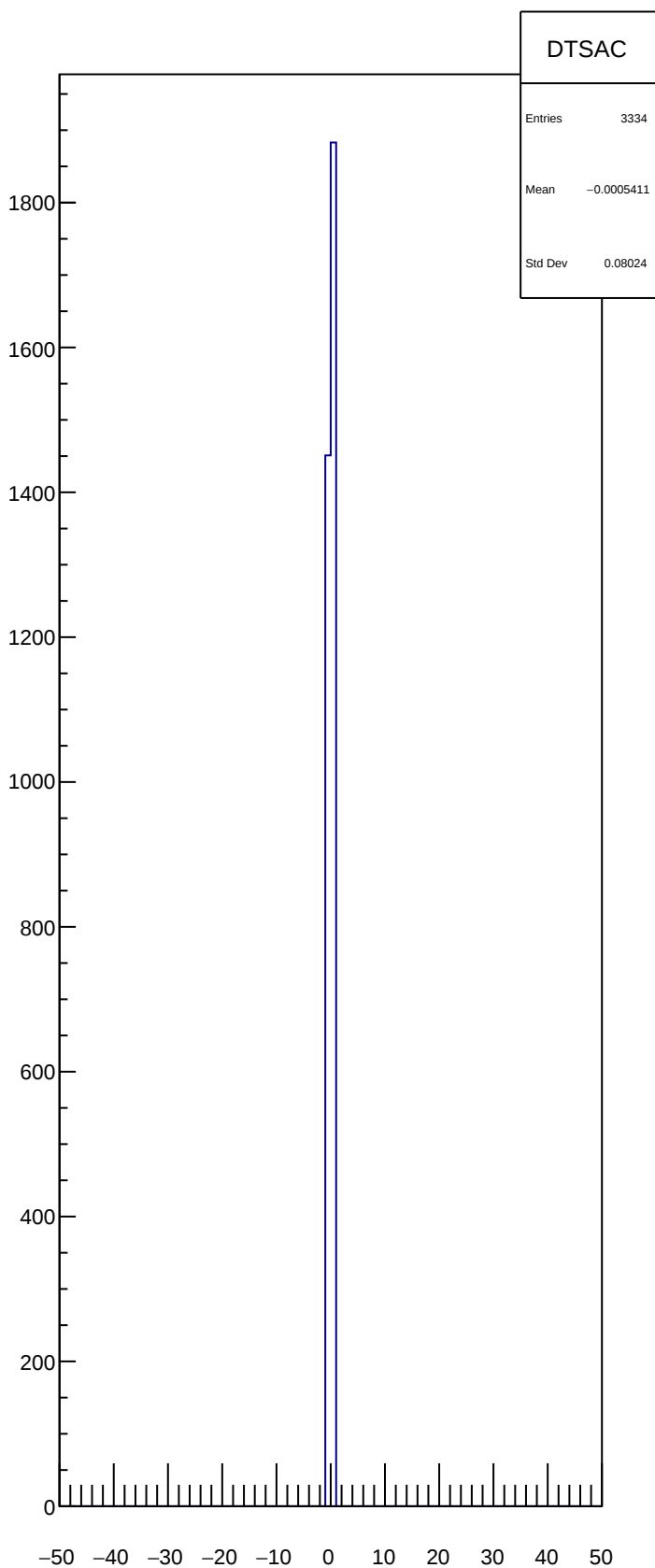
DTSAC
