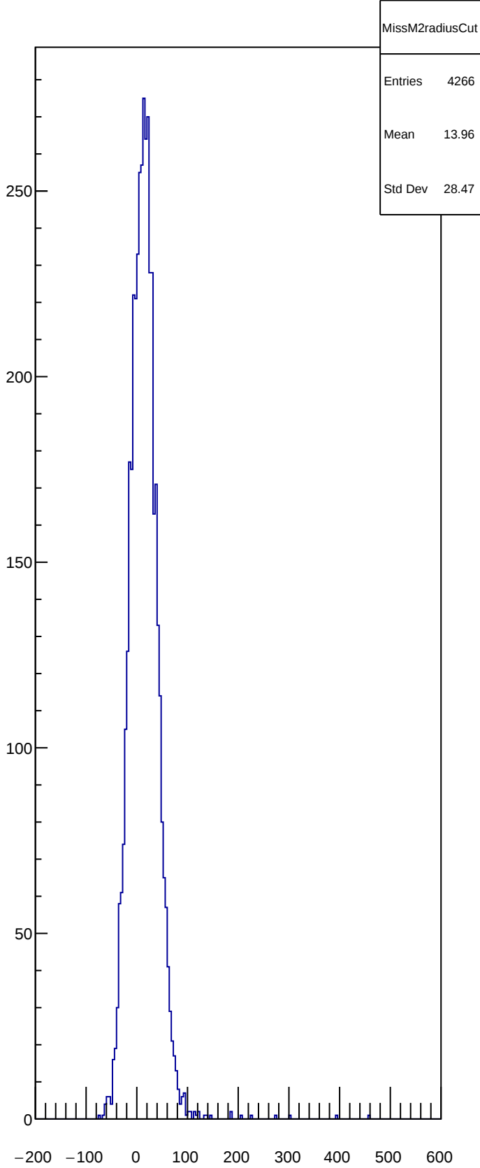
MissM2radiusCut
