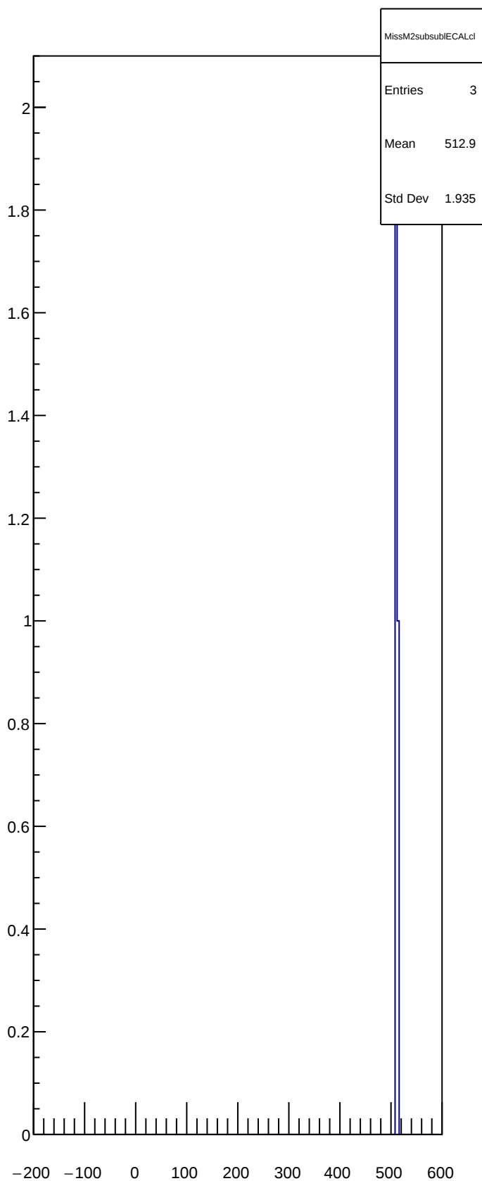
MissM2subsubIECALcl
