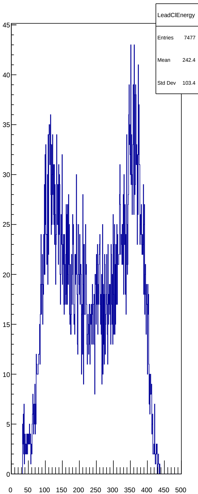
LeadCIEnergy
