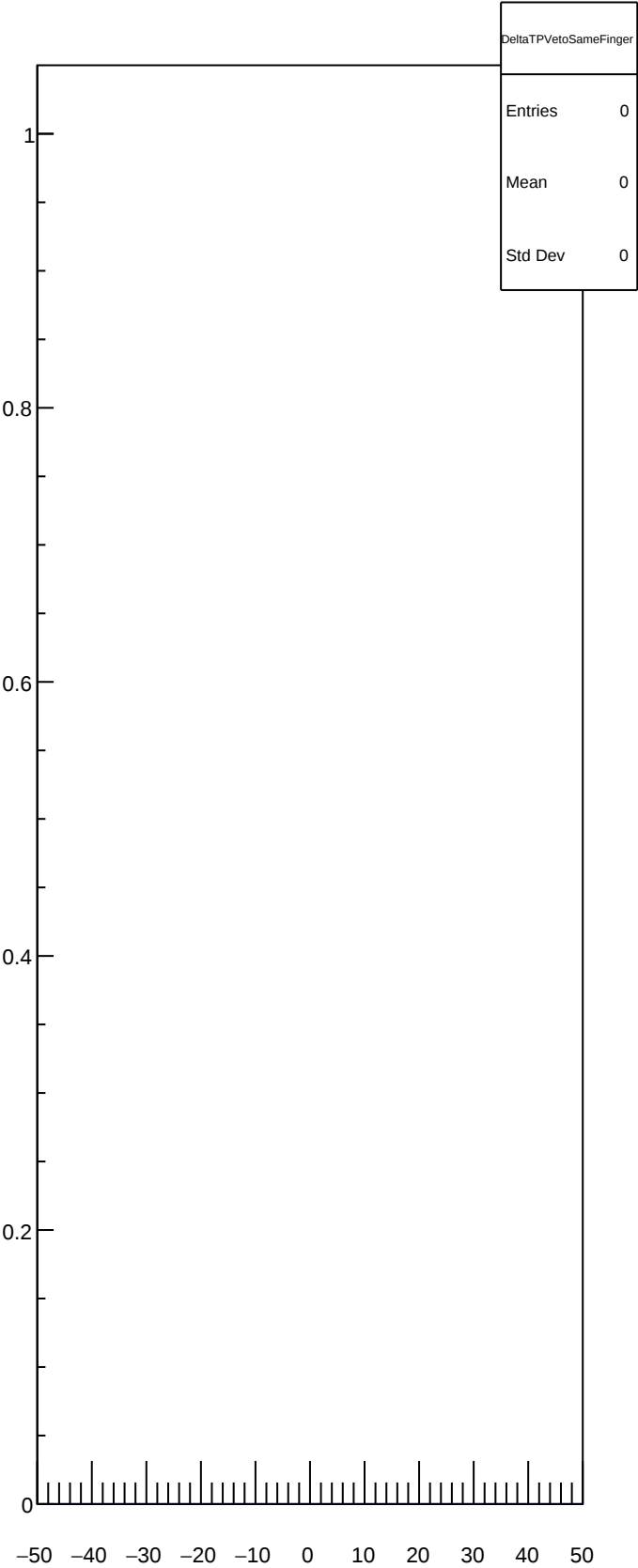
DeltaTPVetoSameFinger
