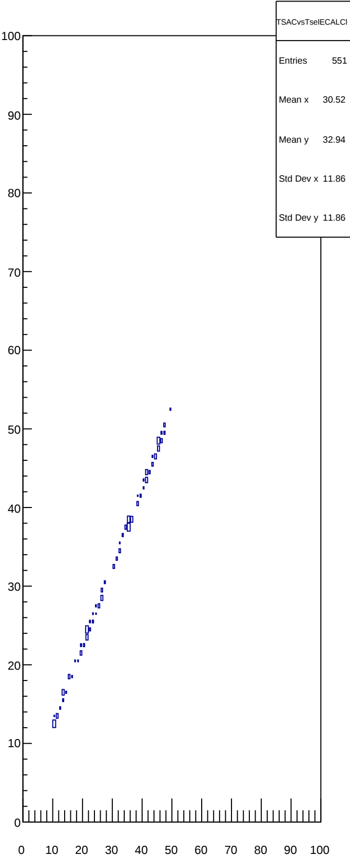
TSACvsTselIECALCI
