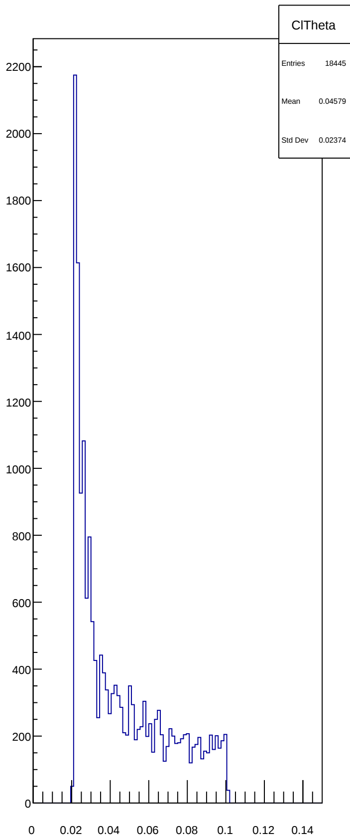
CITheta
