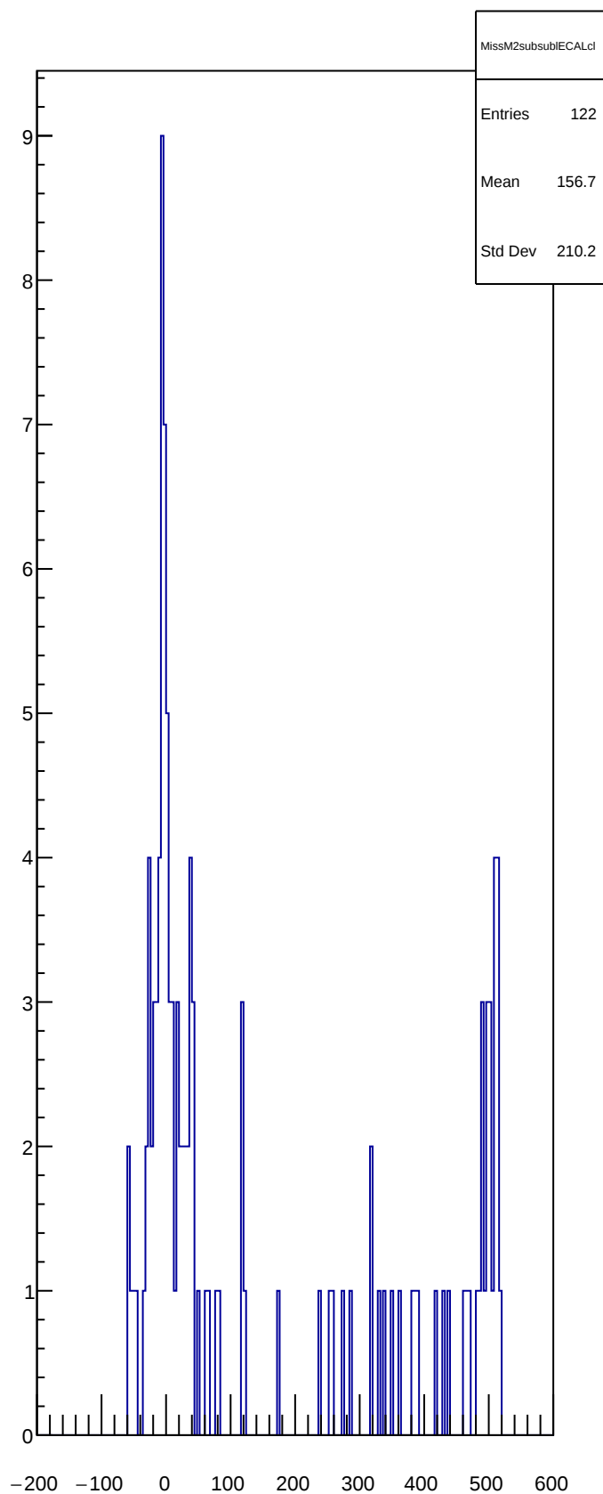
MissM2subsubIECALcl
