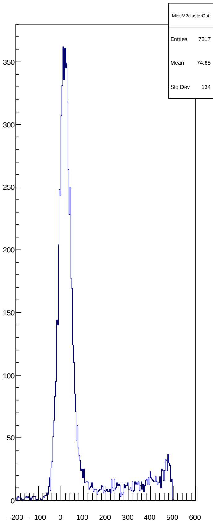
MissM2clusterCut
