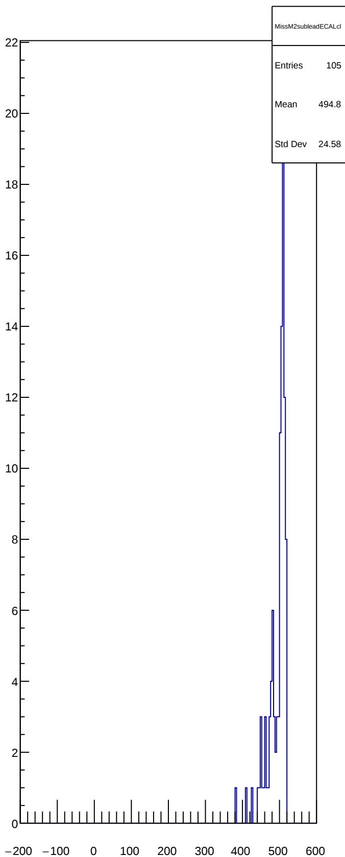
MissM2subleadECALcl
