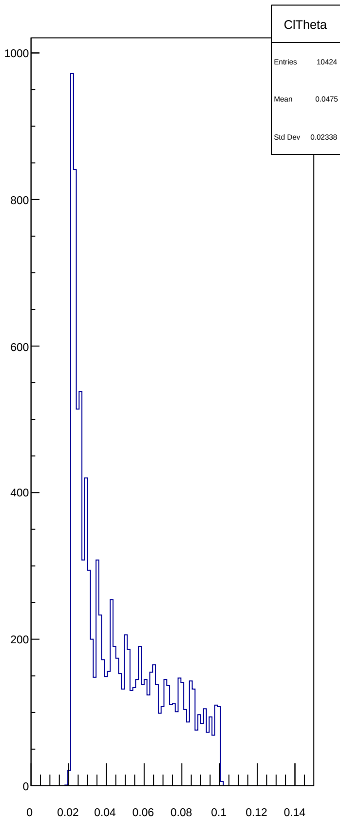
CITheta
