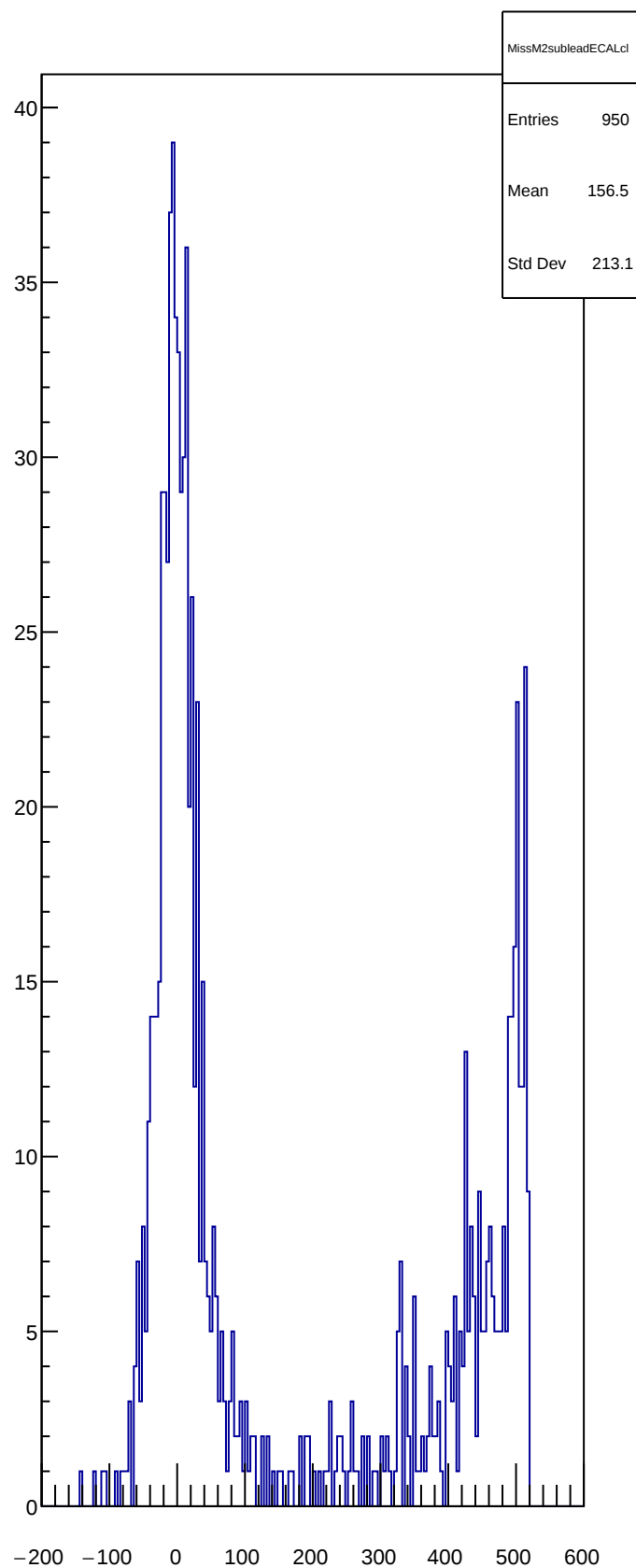
MissM2subleadECALcl
