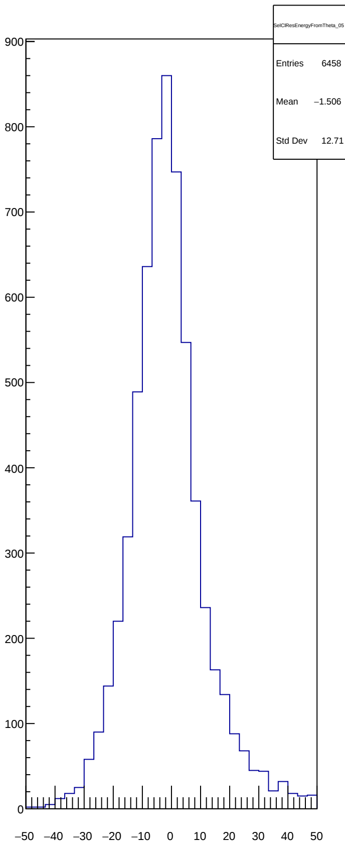
SelClResEnergyFromTheta_05
