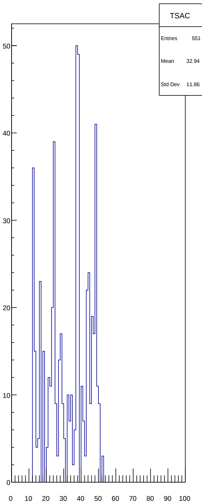
TSAC
