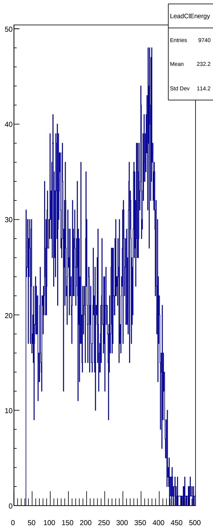
LeadCIEnergy
