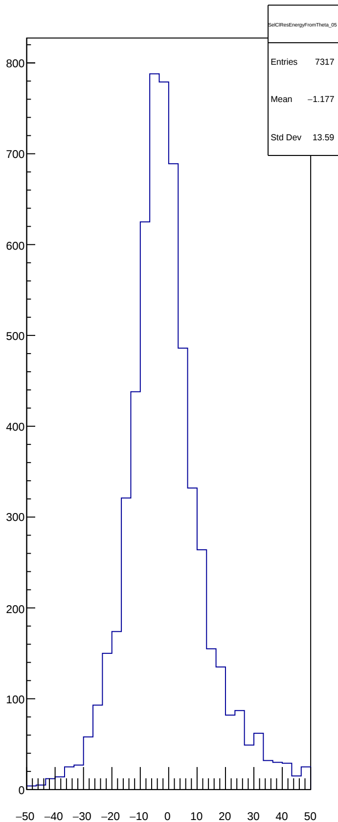
SelClResEnergyFromTheta_05
