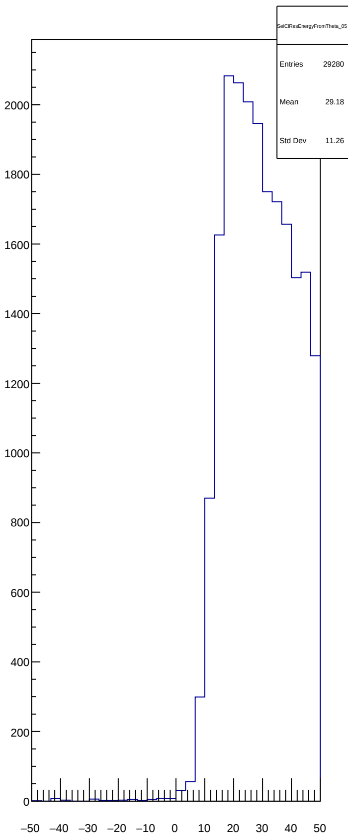
SelClResEnergyFromTheta_05
