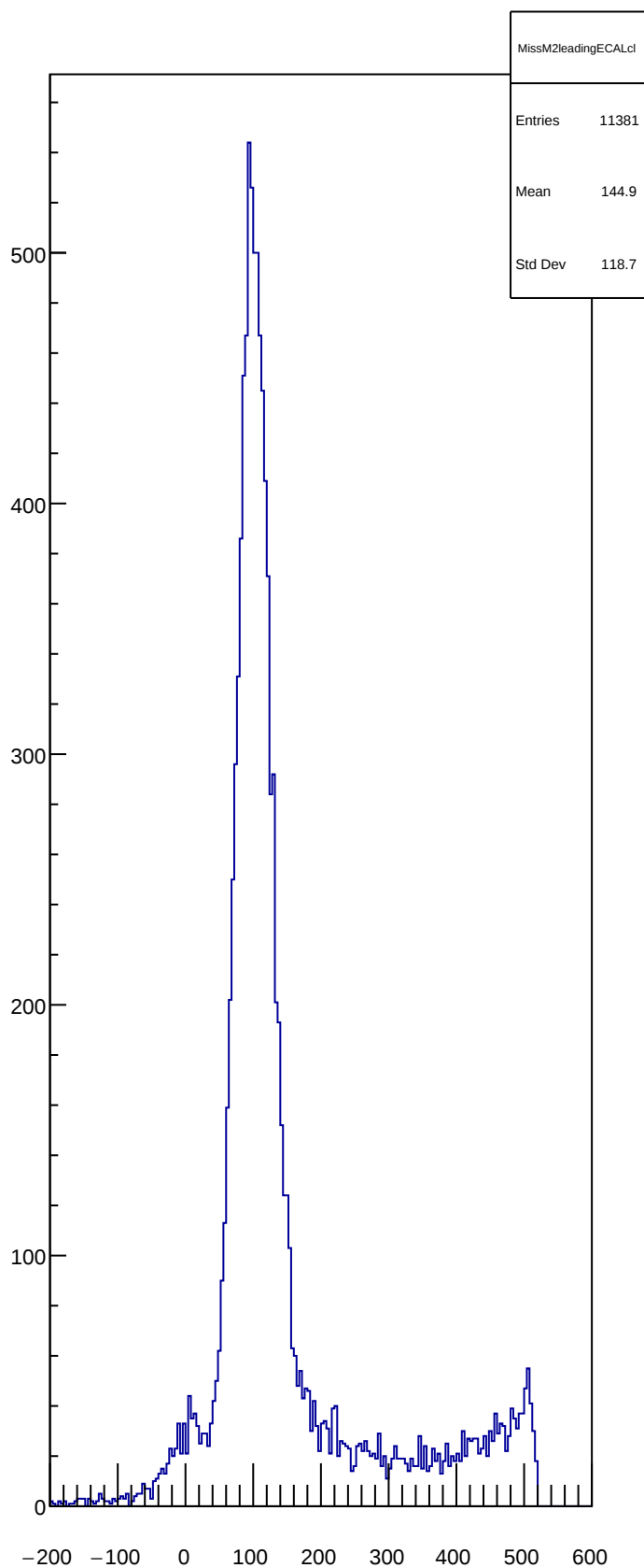
MissM2leadingECALcl
