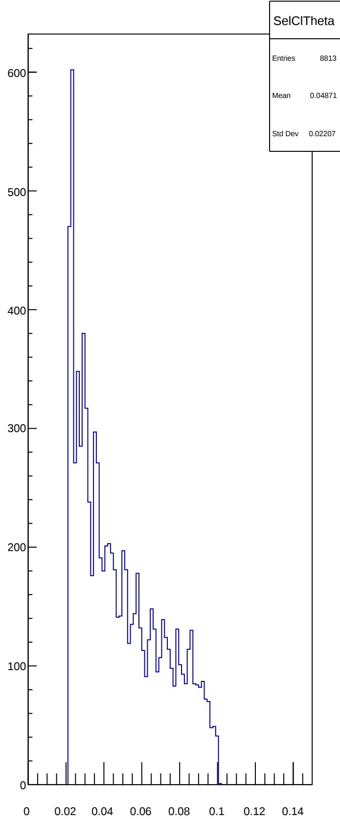
SelCITheta
