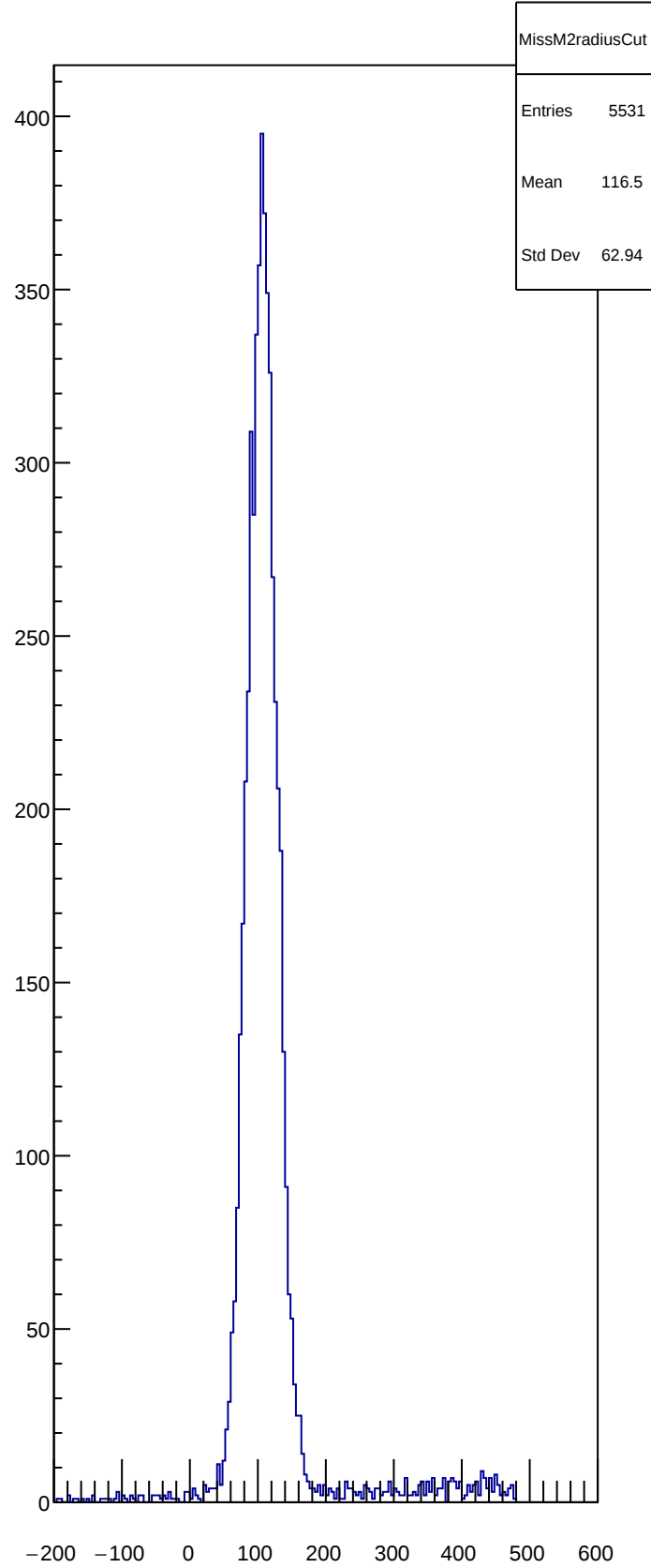
MissM2radiusCut
