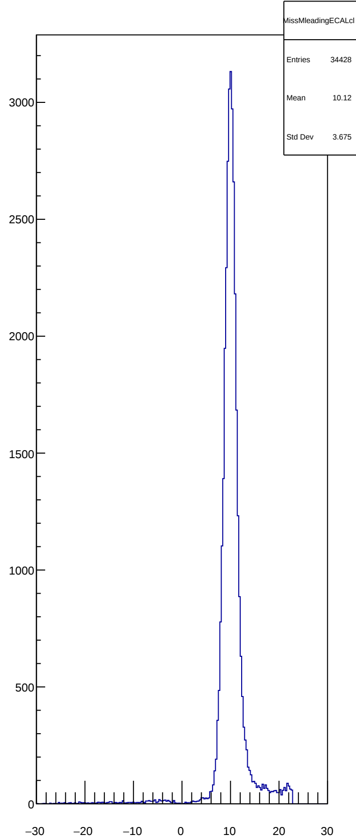
MissMleadingECALcl
