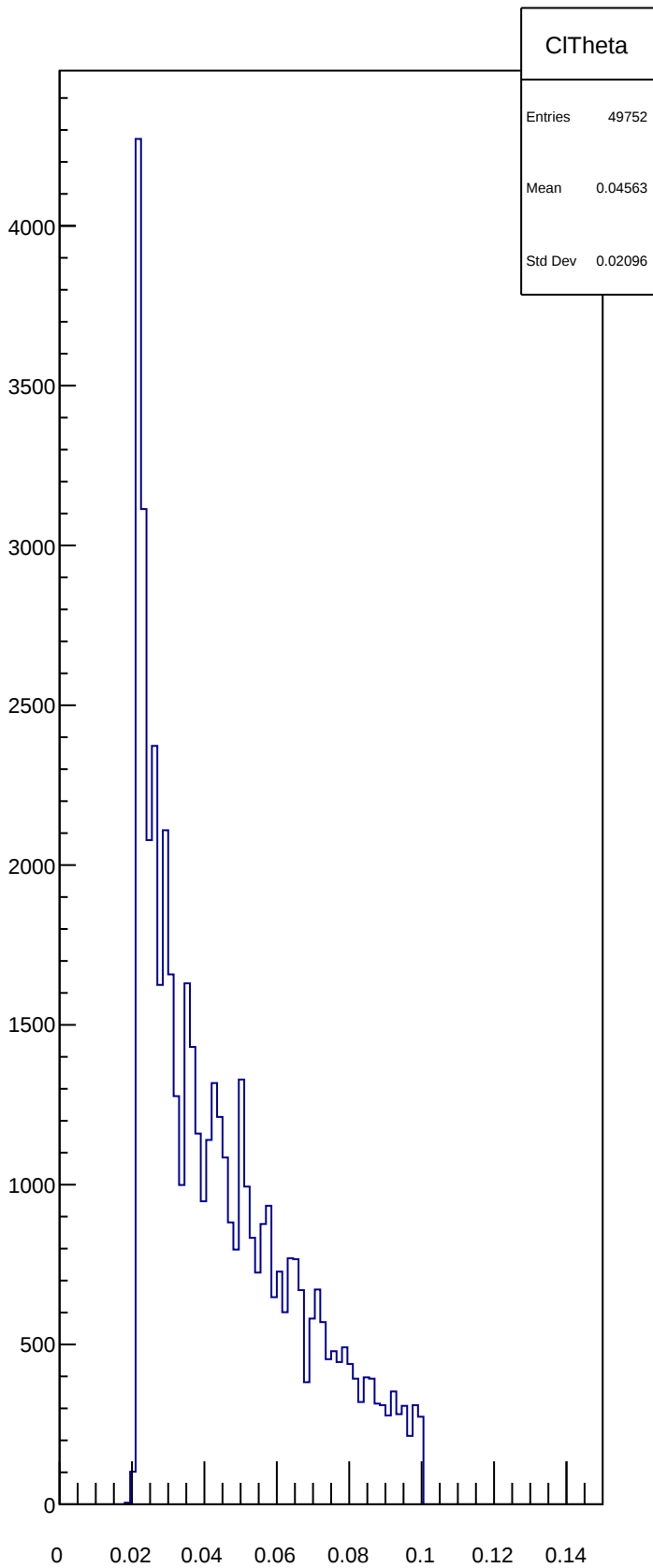
CITheta
