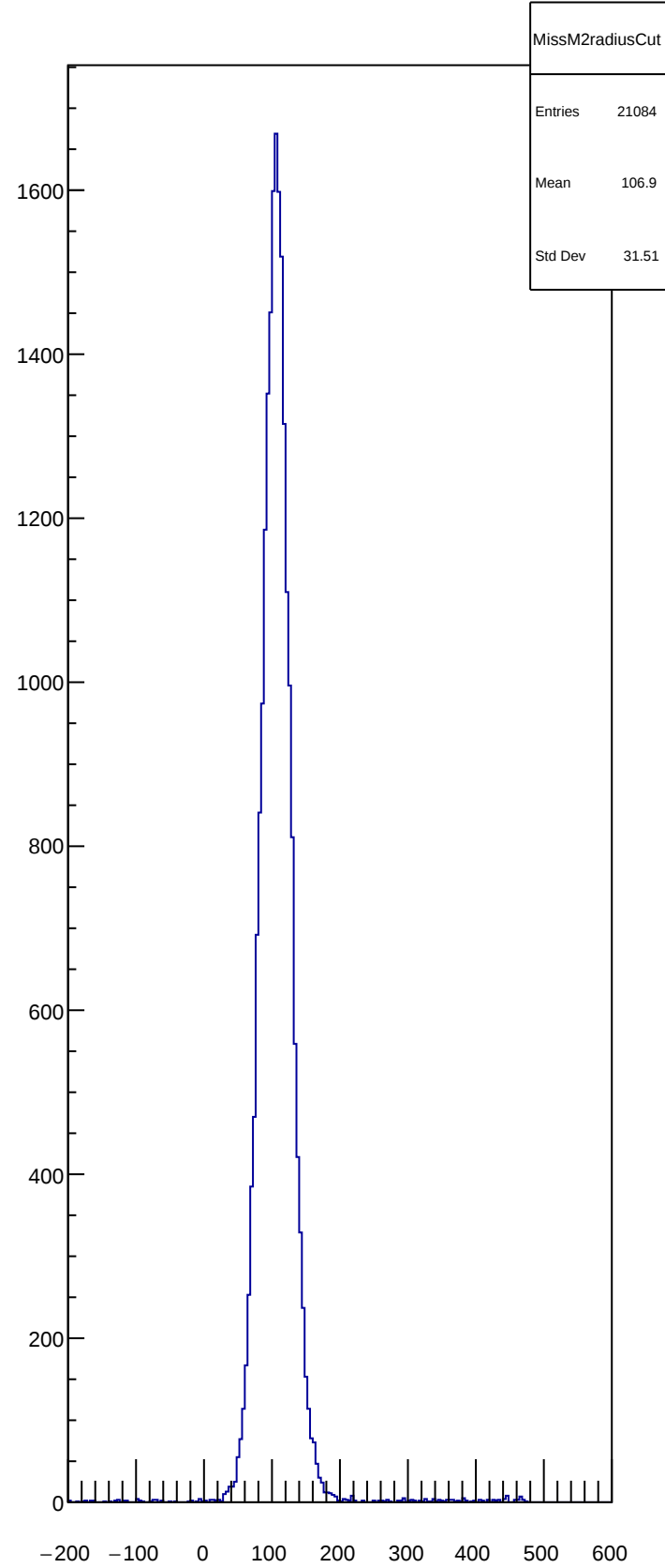
MissM2radiusCut
