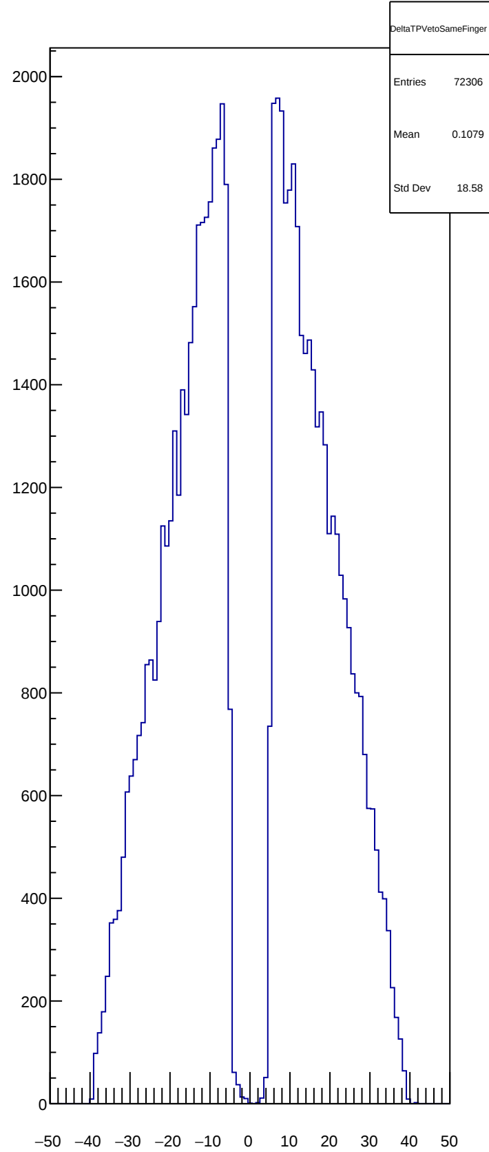
DeltaTPVetoSameFinger
