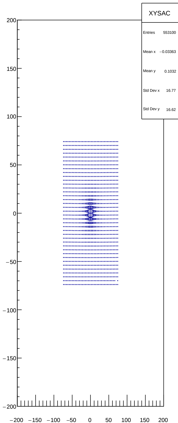
XY SAC
