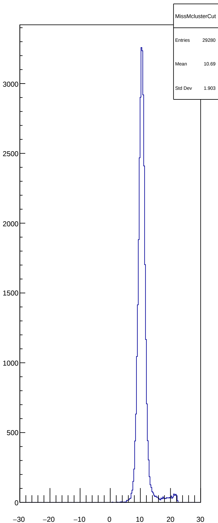
MissMclusterCut
