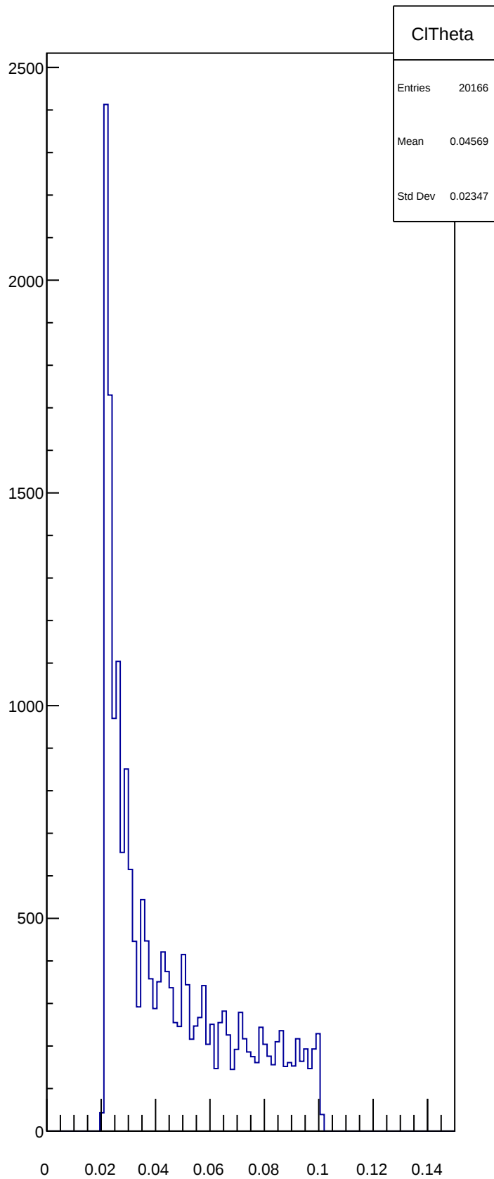
CITheta
