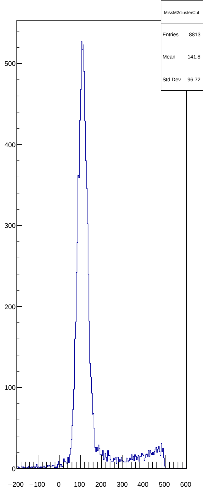
MissM2clusterCut
