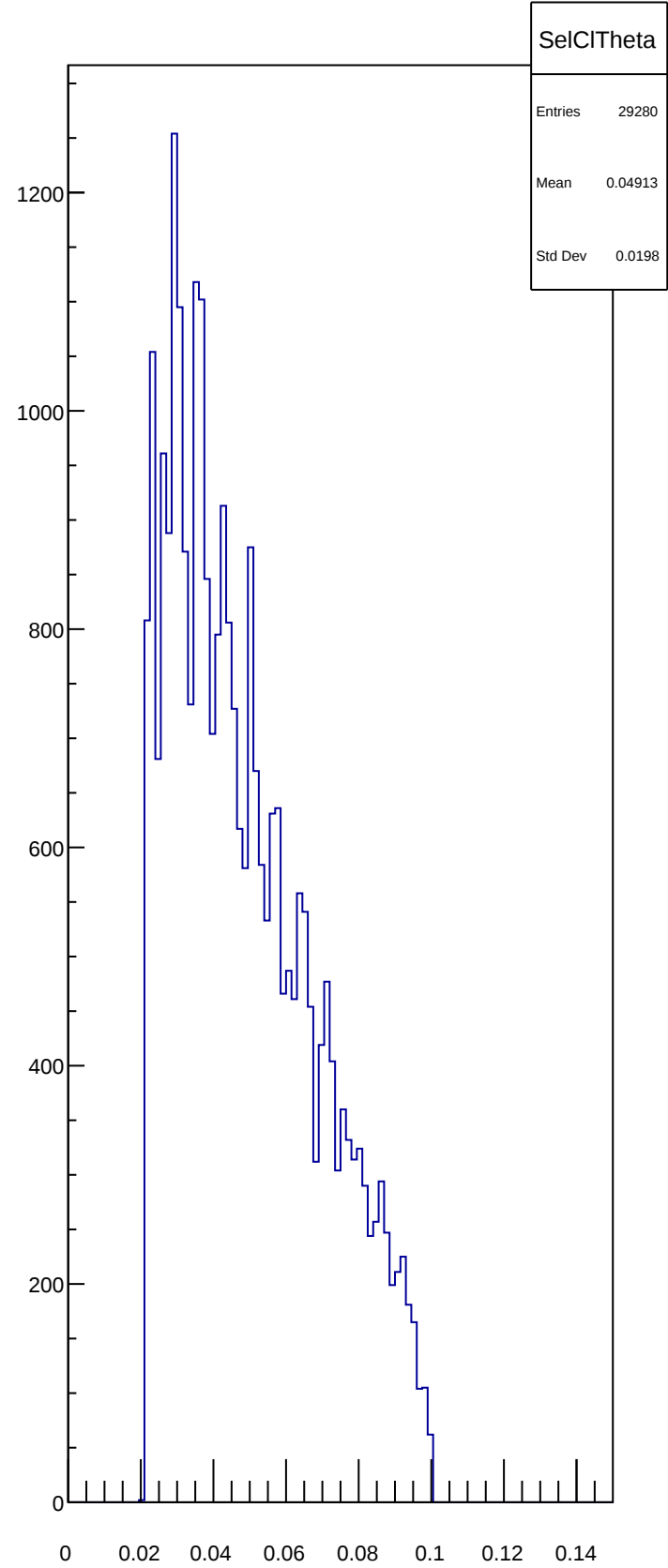
SelCITheta
