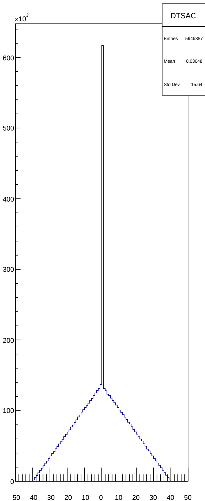
DTSAC
