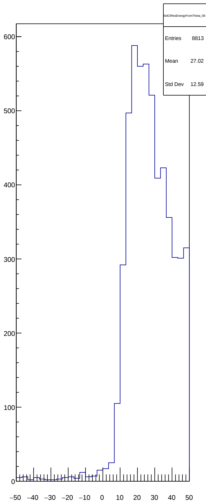
SelClResEnergyFromTheta_05
