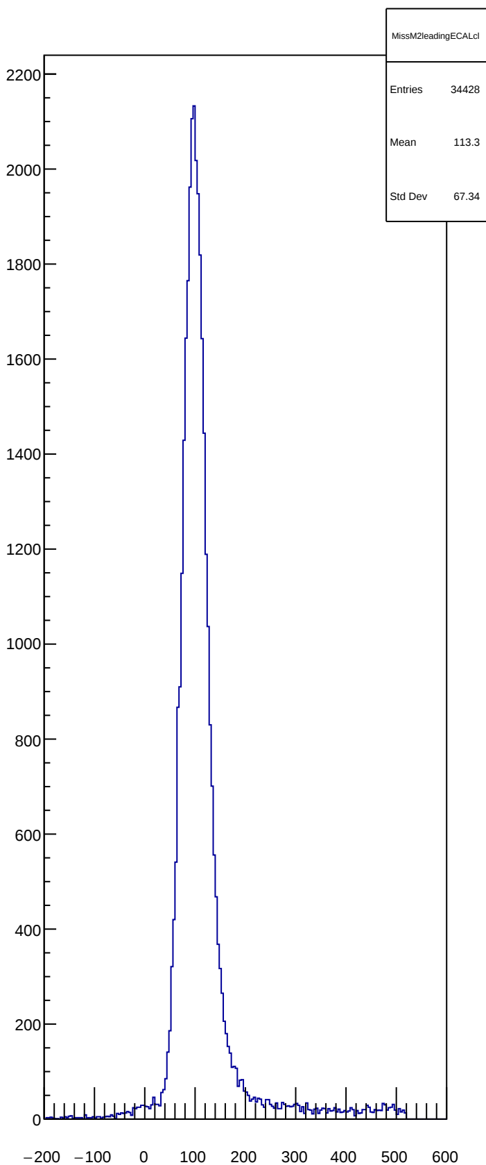
MissM2leadingECALcl
