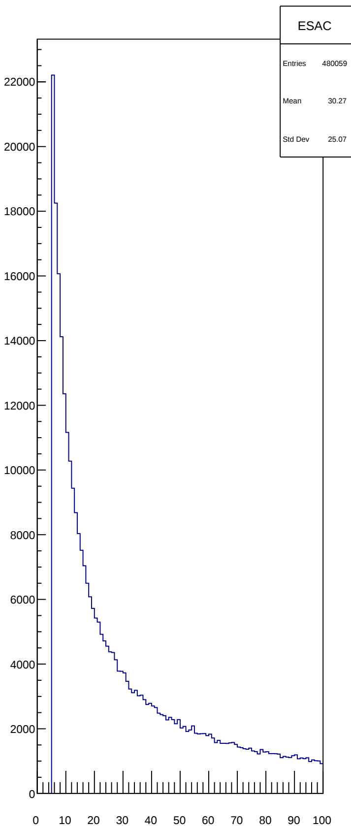
ESAC
