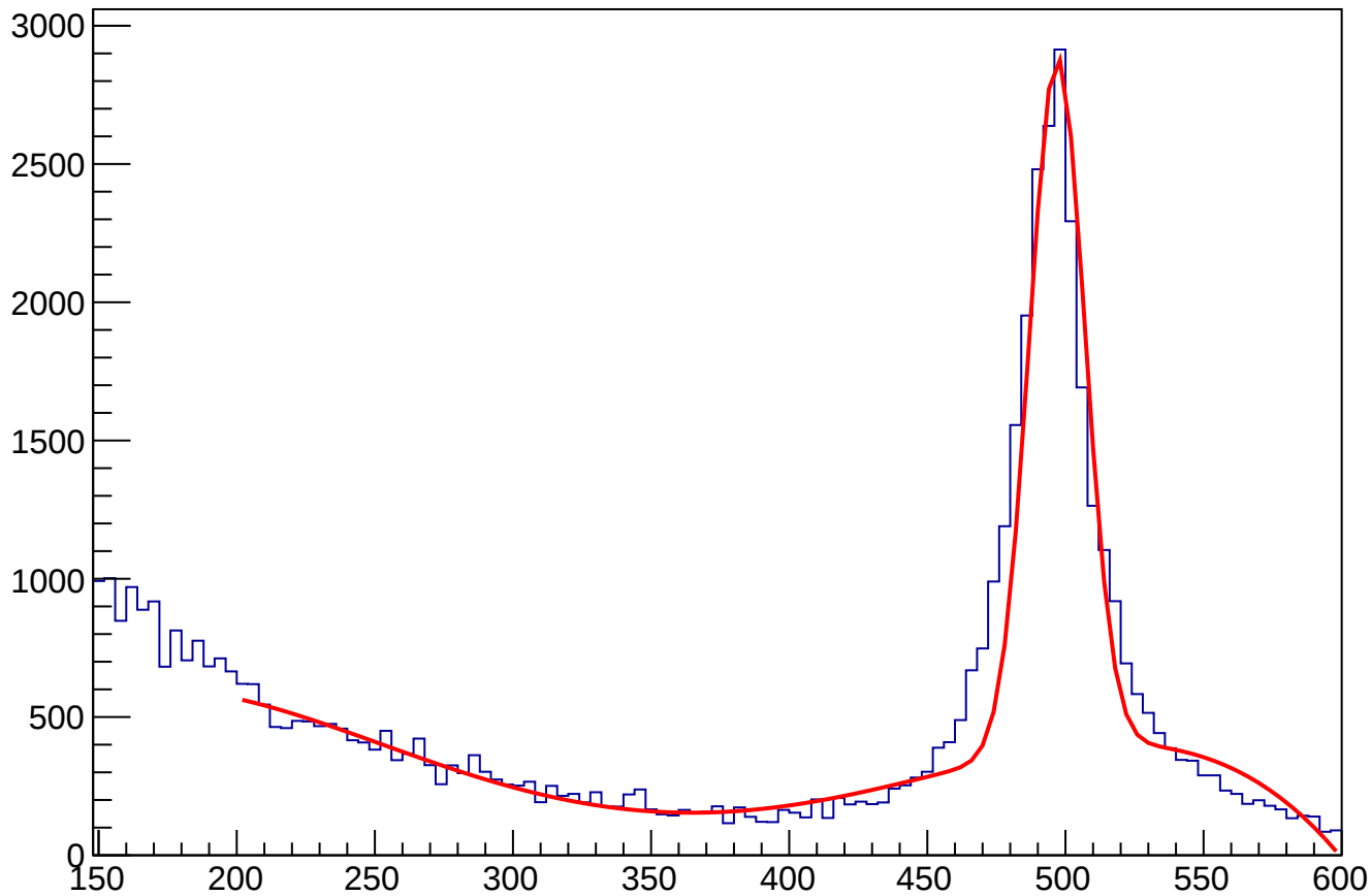
ECAL_gravTwoPhoton1.5ns3cm
