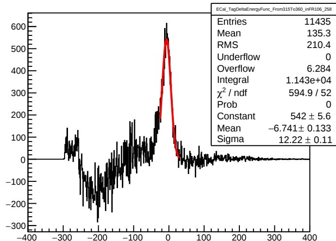
ECal_TagDeltaEnergyFunc_From315To360_inFR106_258
