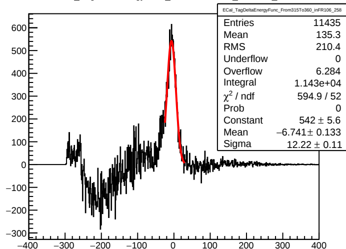
ECal_TagDeltaEnergyFunc_From315To360_inFR106_258
