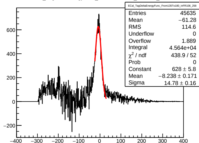
ECal_TagDeltaEnergyFunc_From135To180_inFR106_258
