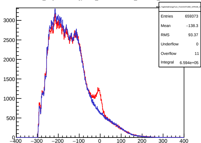
ECal_TagDeltaEnergyFunc_From315To360_inFR106_258
