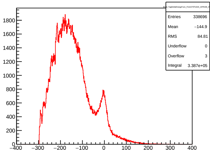
ECal_TagDeltaEnergyFunc_From270To315_inFR106_258
