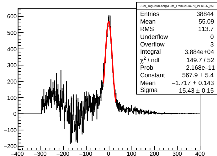
ECal_TagDeltaEnergyFunc_From225To270_inFR106_258
