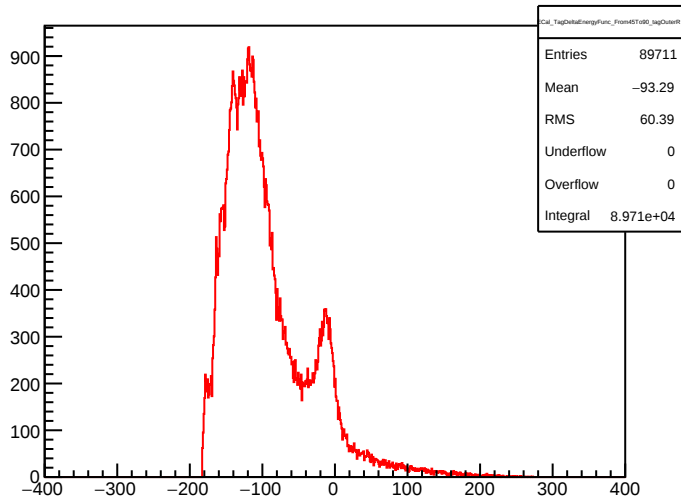
ECal_TagDeltaEnergyFunc_From45To90_tagOuterR
