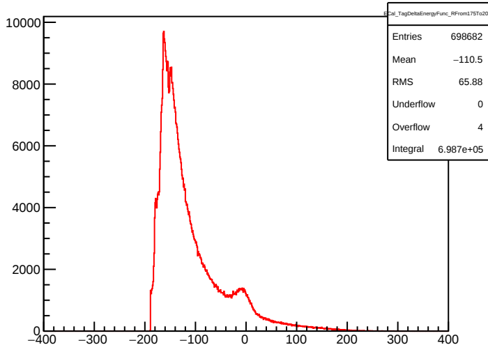
ECal_TagDeltaEnergyFunc_RFrom175To200
