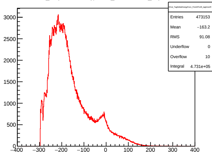
ECal_TagDeltaEnergyFunc_From0To45_tagInnerR
