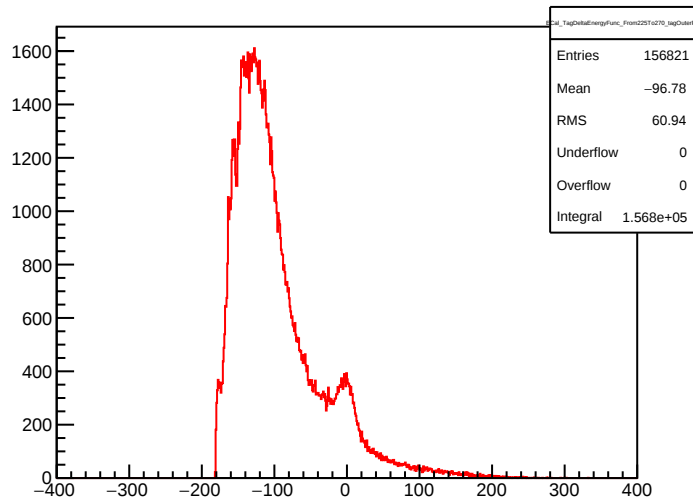
ECal_TagDeltaEnergyFunc_From225To270_tagOuterR
