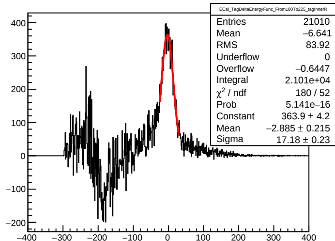
ECal_TagDeltaEnergyFunc_From180To225_tagInnerR
