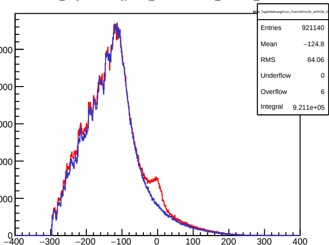
ECal_TagDeltaEnergyFunc_From180To225_inFR106_258
