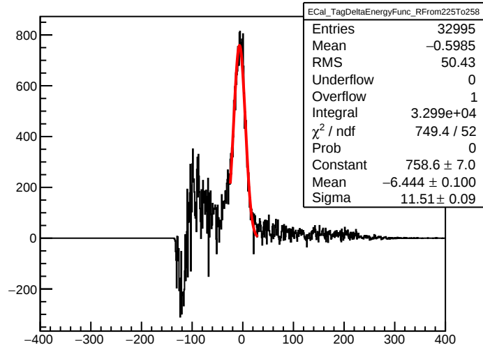
ECal_TagDeltaEnergyFunc_RFrom225To258
