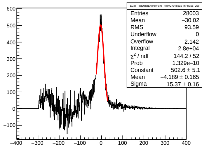
ECal_TagDeltaEnergyFunc_From270To315_inFR106_258
