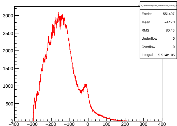
ECal_TagDeltaEnergyFunc_From90To135_inFR106_258
