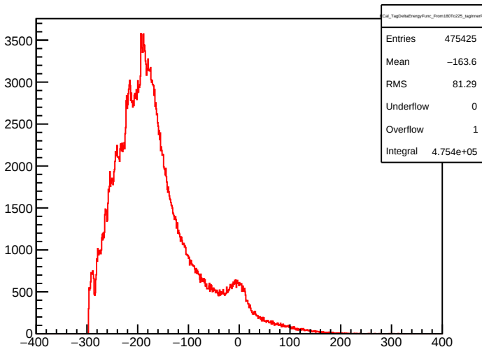
ECal_TagDeltaEnergyFunc_From180To225_tagInnerR
