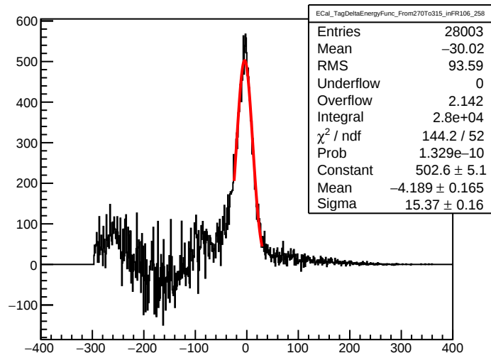
ECal_TagDeltaEnergyFunc_From270To315_inFR106_258
