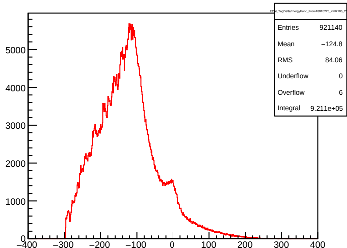
ECal_TagDeltaEnergyFunc_From180To225_inFR106_258
