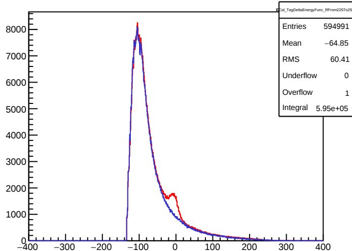
ECal_TagDeltaEnergyFunc_RFrom225To258
