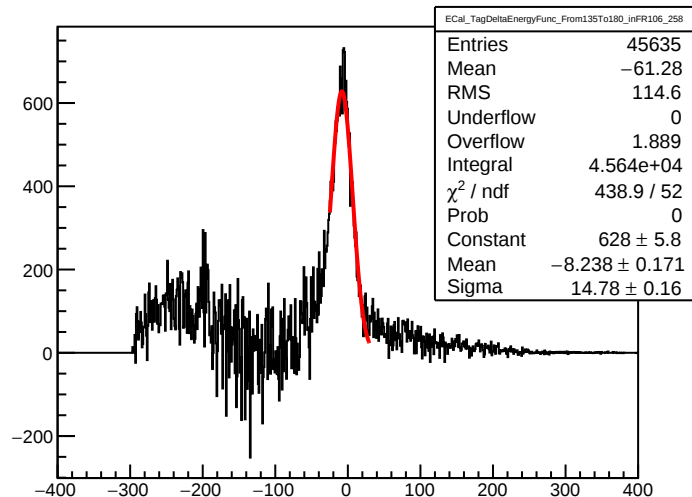
ECal_TagDeltaEnergyFunc_From135To180_inFR106_258
