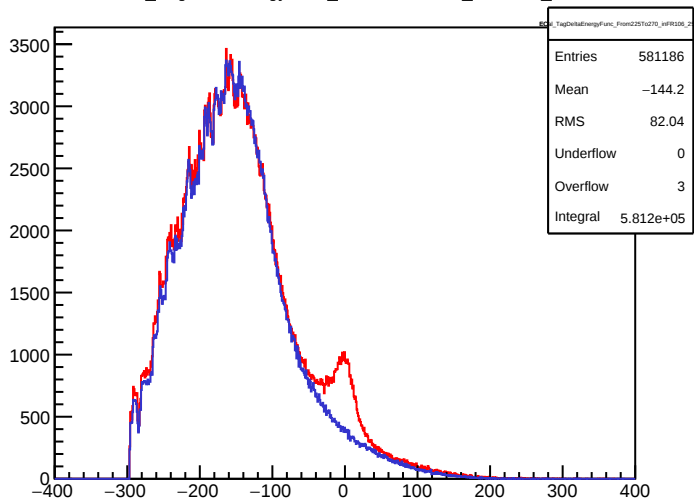
ECal_TagDeltaEnergyFunc_From225To270_inFR106_258
