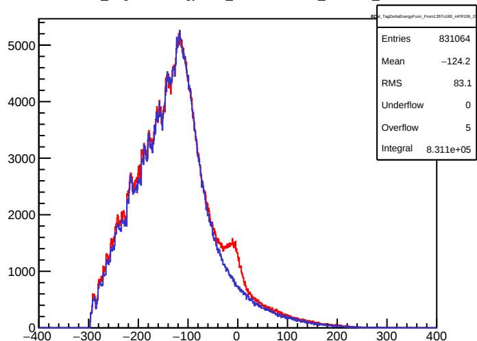
ECal_TagDeltaEnergyFunc_From135To180_inFR106_258
