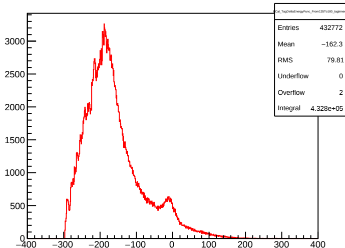
ECal_TagDeltaEnergyFunc_From135To180_tagInnerR
