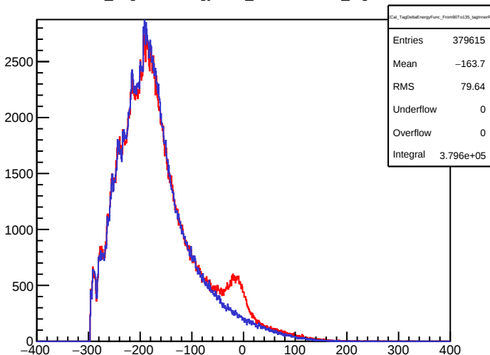
ECal_TagDeltaEnergyFunc_From90To135_tagInnerR
