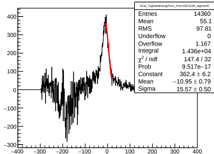
ECal_TagDeltaEnergyFunc_From135To180_tagInnerR
