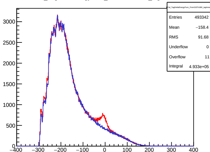
ECal_TagDeltaEnergyFunc_From315To360_tagInnerR
