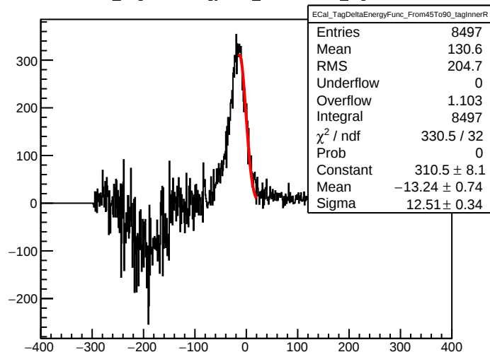
ECal_TagDeltaEnergyFunc_From45To90_tagInnerR
