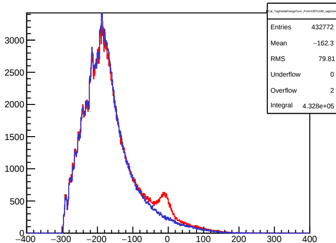
ECal_TagDeltaEnergyFunc_From135To180_tagInnerR
