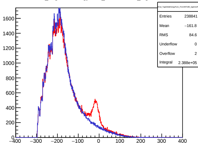
ECal_TagDeltaEnergyFunc_From45To90_tagInnerR
