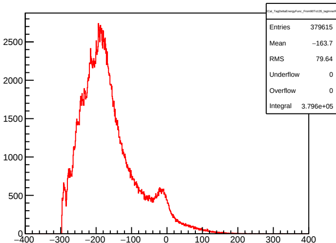
ECal_TagDeltaEnergyFunc_From90To135_tagInnerR
