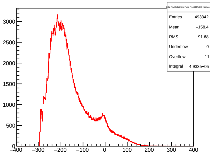
ECal_TagDeltaEnergyFunc_From315To360_tagInnerR
